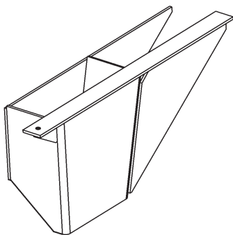
Soporte de montaje izquierdo, galvanizado (GPT) N/P 282666-01G Cant. 1
