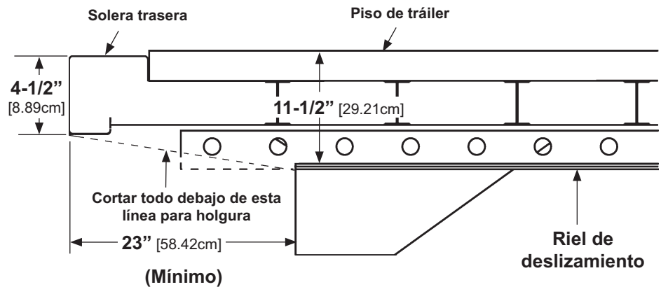
Cortar chasis para tráiler estándar FIG. 3-1
