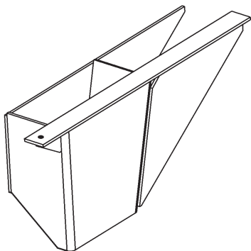
Soporte de montaje izquierdo, galvanizado (GPT) N/P 282960-01G Cant. 1
