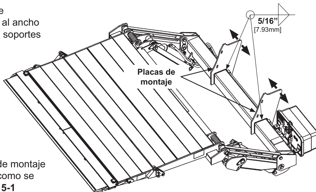
Ejemplo para mover placas de montaje pintadas en el marco principal y soldar en su lugar FIG. 5-1
