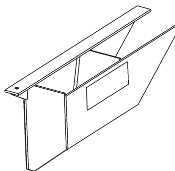
Soporte de montaje derecho, galvanizado (GPT) N/P 282666-02G Cant. 1
