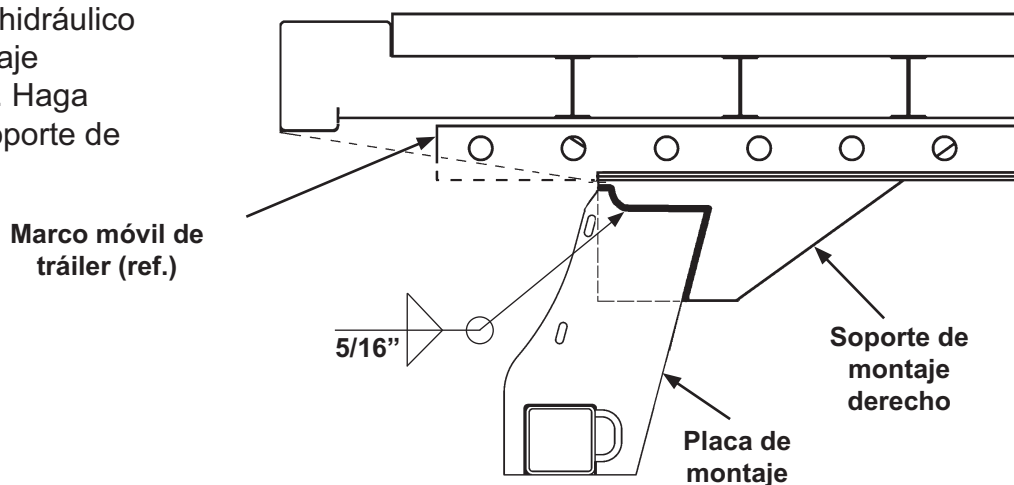
Ejemplo para soldar placas de montaje a soporte de montaje en el tráiler (se muestra lado derecho) FIG. 5-2
