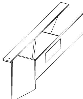
Soporte de montaje derecho, galvanizado (GPT) N/P 282960-02G Cant. 1
