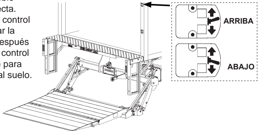
VERIFICAR INTERRUPTOR DE CONTROL DOBLE FIG. 16-2
