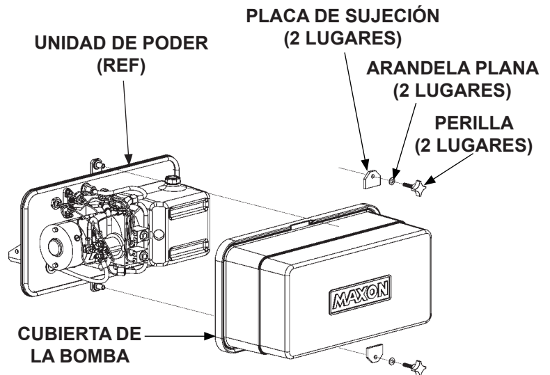
ATORNILLAR/DESATORNILLAR LA CUBIERTA DE LA BOMBA FIG. 14-2
