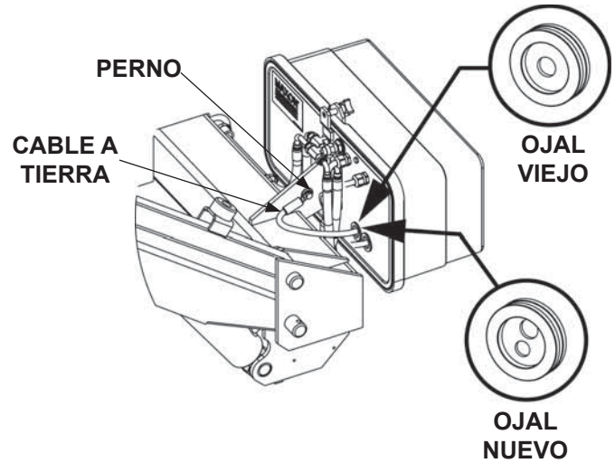
REEMPLAZAR OJAL FIG. 14-1
