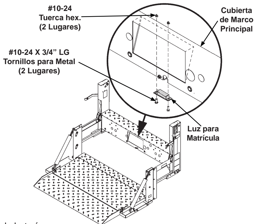
Instalar Luces para Matrícula En Elevador C2 FIG. 4-2
