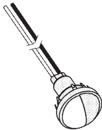
Luz para Matrícula (Elevadores C1) N/P 289549-01 Cant. 2
