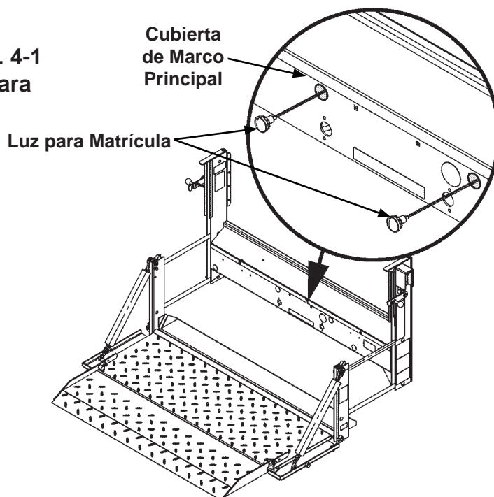
Instalar Luces para Matrícula En Elevador C1 FIG. 4-1
