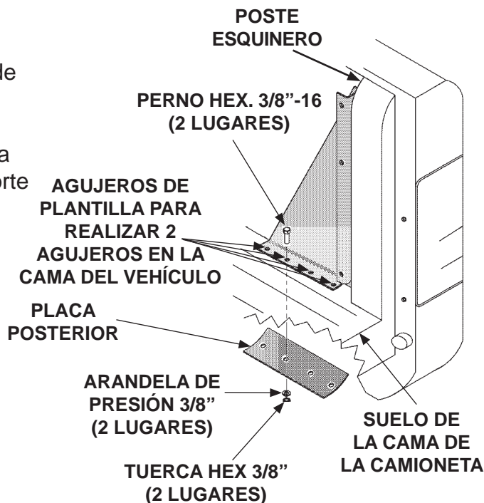
ATORNILLAR SOPORTE DE MONTAJE DERECHO A LA CAMA DE LA CAMIONETA (NO SE MUESTRA ELEVADOR) FIG. 32-1
