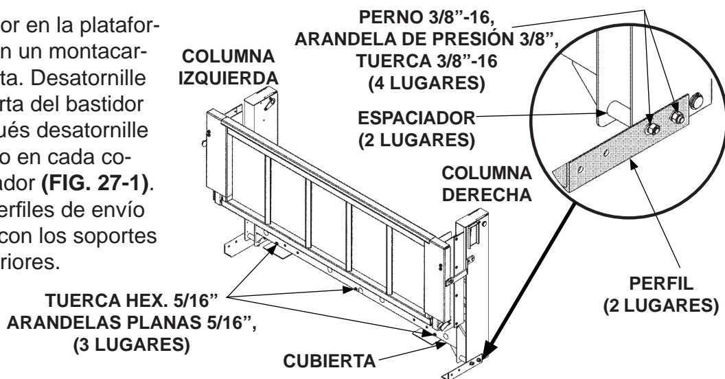
RETIRAR PERFILES DE ENVÍO FIG. 27-1
