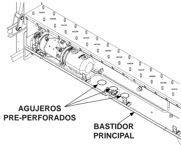
ABRIR LOS AGUJEROS PRE-PERFORADOS DE LA CARCASA DEL BASTIDOR PRINCIPAL FIG. 28-1
