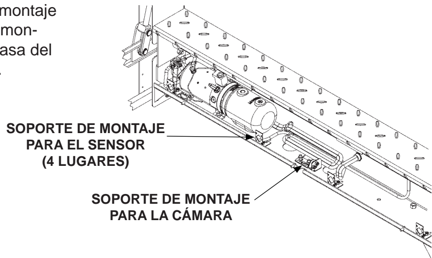
UBICACIÓN DEL SOPORTE DE LA CÁMARA Y DEL SENSOR FIG. 38-1
