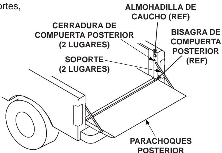
RETIRAR COMPUERTA POSTERIOR Y SOPORTES FIG. 30-1
