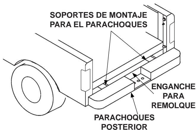
RETIRAR PARACHOQUES POSTERIOR FIG. 30-2
