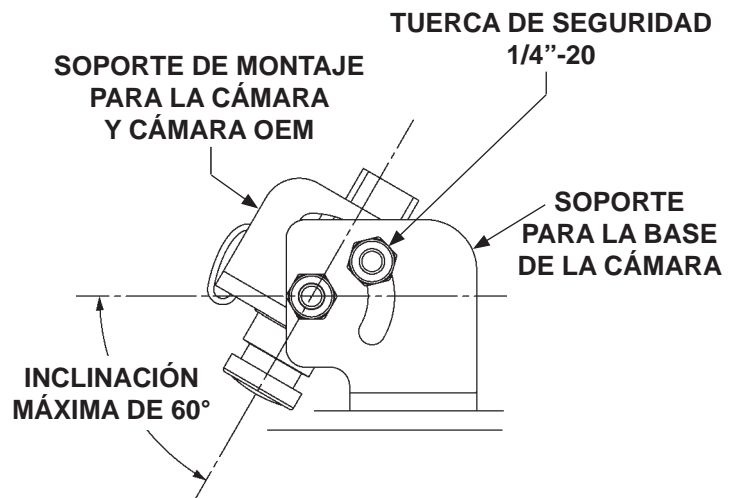
AJUSTAR EL ÁNGULO DE LA CÁMARA FIG. 39-1
