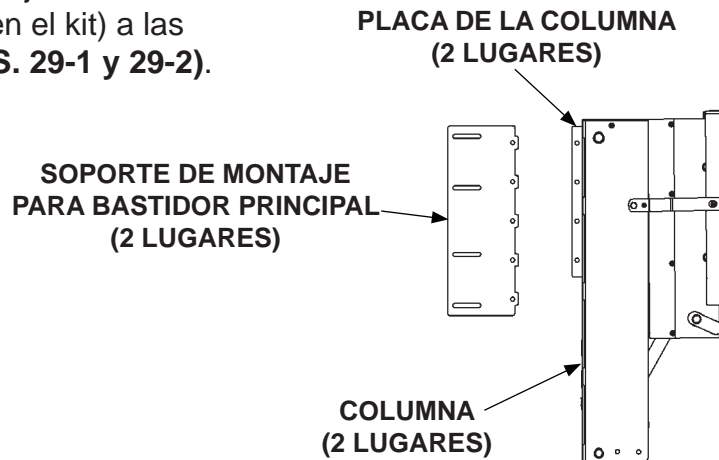
SE MUESTRA ELEVADOR C2 CON SOPORTES DE MONTAJE PARA ATORNILLARSE EN EL BASTIDOR PRINCIPAL FIG. 29-1
