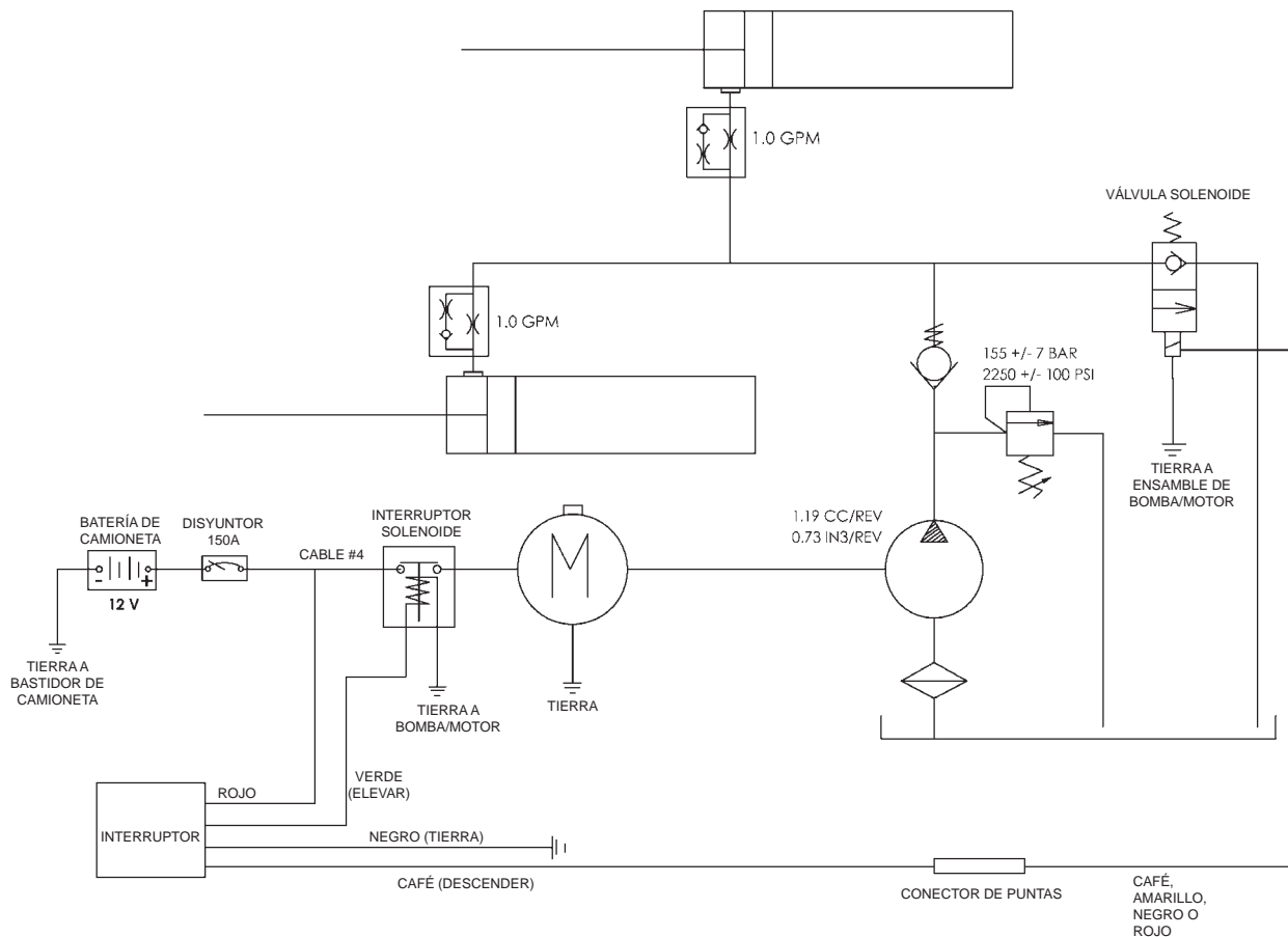
DIAGRAMA DE SISTEMAS ELÉCTRICOS E HIDRÁULICOS PARA ELEVADOR C2 FIG. 36-1
