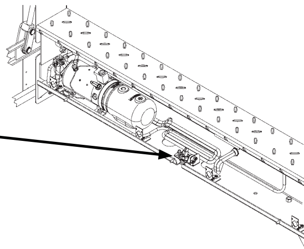
AGREGAR LA CÁMARA AL SOPORTE DE MONTAJE FIG. 38-2
