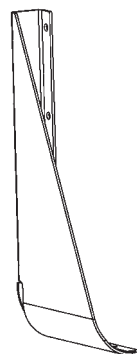
SOPORTE PARA MONTAJE, DERECHO N/P 295039-02G CANT. 1
