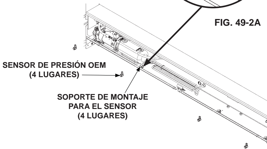
INSTALAR SENSORES (SI SE EQUIPA) FIG. 49-2
