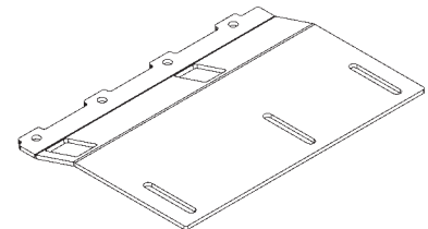
SOPORTE DERECHO DE MONTAJE DEL BASTIDOR PRINCIPAL (GALVANIZADO) N/P 299929-02G CANT. 1
