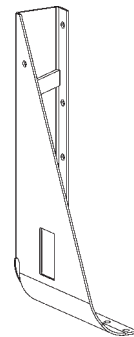
SOPORTE DERECHO DE MONTAJE (GALVANIZADO) N/P 299943-02G CANT. 1
