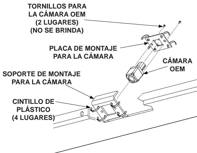
AGREGAR LA CÁMARA A LA PLACA DE MONTAJE Y EL SOPORTE DE MONTAJE FIG. 48-2
