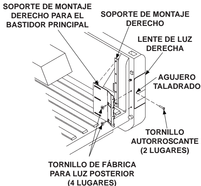
MODIFICAR MONTAJE DE LUZ POSTERIOR FIG. 39-1
