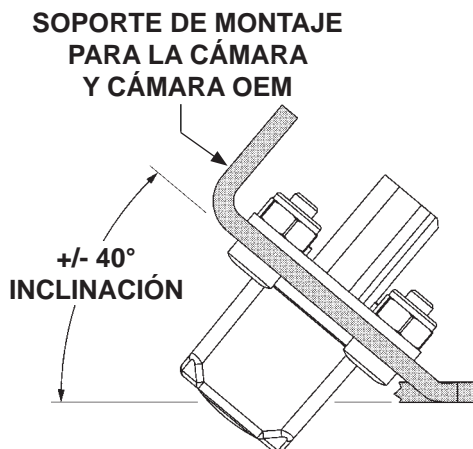
AJUSTAR EL ÁNGULO DE LA CÁMARA FIG. 49-1
