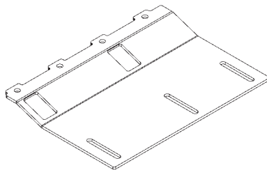
SOPORTE IZQUIERDO DE MONTAJE DEL BASTIDOR PRINCIPAL (GALVANIZADO) N/P 299929-01G CANT. 1
