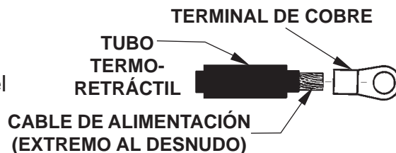
COLOCAR TERMINAL DE COBRE Y TUBO TERMORETRÁCTIL EN CABLE DE ALIMENTACIÓN FIG. 45-2
