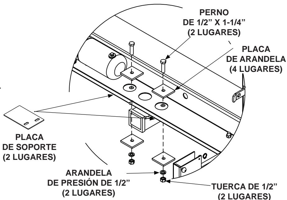
INSTALAR PLACA DE ARANDELA EN ENGANCHE CLASE 5 FIG. 52-2
