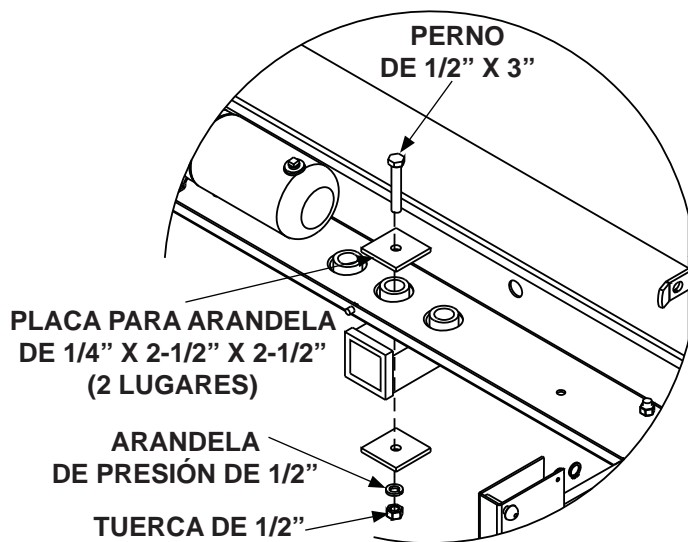
INSTALAR PLACA DE ARANDELA EN ENGANCHE CLASE 4 FIG. 52-1
