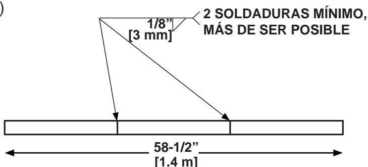
POSICIÓN Y SOLDADURAS PARA TIRA DE RELLENO FIG. 40-1
