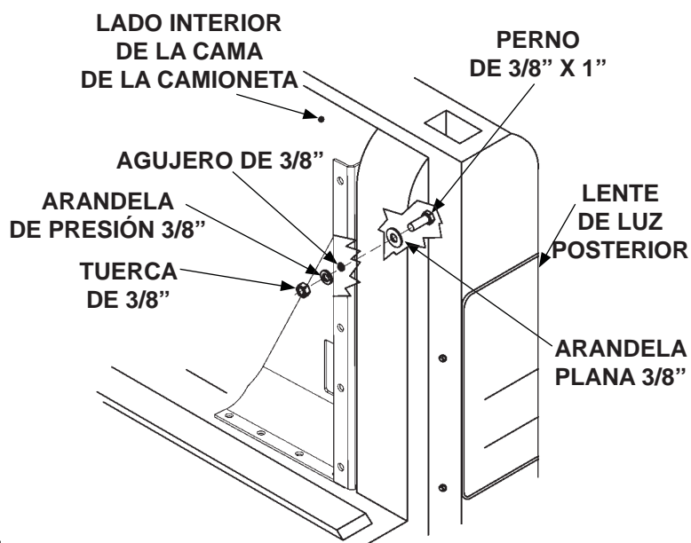
AJUSTAR SOPORTE A LA CAMA DE LA CAMIONETA (SE MUESTRA LADO DERECHO) FIG. 42-1
