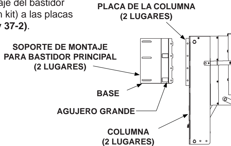
SE MUESTRA ELEVADOR C2 CON SOPORTES PARA ATORNILLAR EN EL BASTIDOR PRINCIPAL FIG. 37-1
