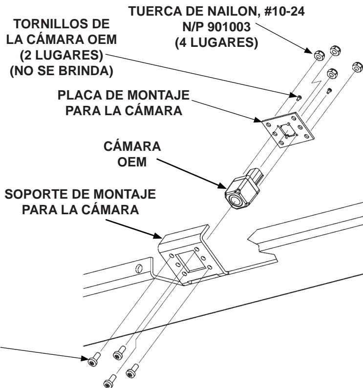
AGREGAR LA CÁMARA A LA PLACA DE MONTAJE Y EL SOPORTE DE MONTAJE FIG. 48-1
