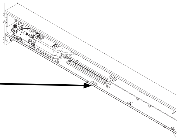
AJUSTAR EL SOPORTE DE LA CÁMARA FIG. 47-2
