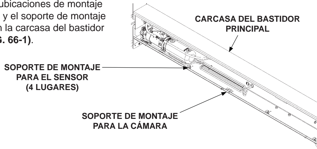
UBICACIÓN DEL SOPORTE DE LA CÁMARA Y DEL SENSOR FIG. 66-1
