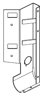
SOPORTE DE MONTAJE DERECHO N/P 209329-02 (PINTADO) N/P 209329-02G (GALVANIZADO) CANT. 1
