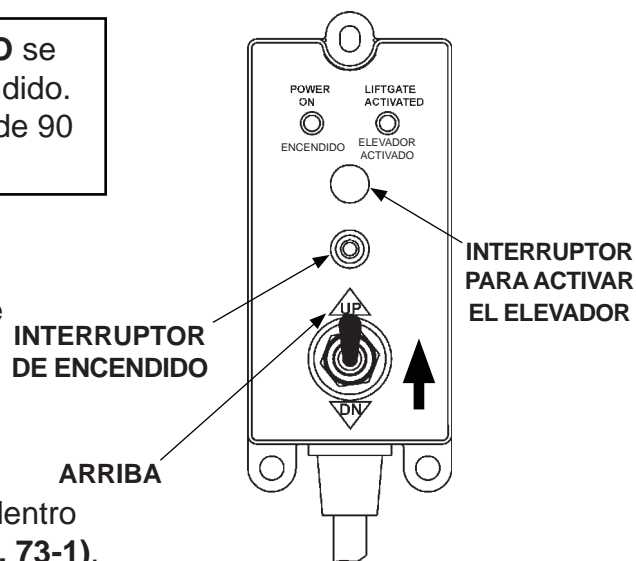
VERIFICAR OPERACIÓN DEL INTERRUPTOR DE CONTROL Y ELEVAR LA PLATAFORMA FIG. 73-1
