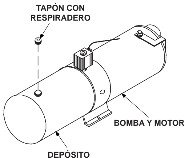
INSTALAR TAPÓN DE VENTILACIÓN EN EL DEPÓSITO DE LA BOMBA FIG. 71-1
