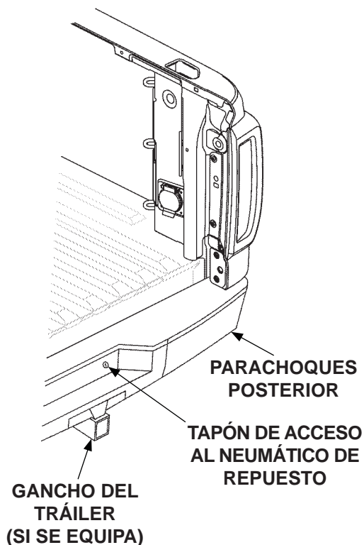
RETIRAR LA COMPUERTA POSTERIOR Y EL PARACHOQUES POSTERIOR FIG. 51-1
