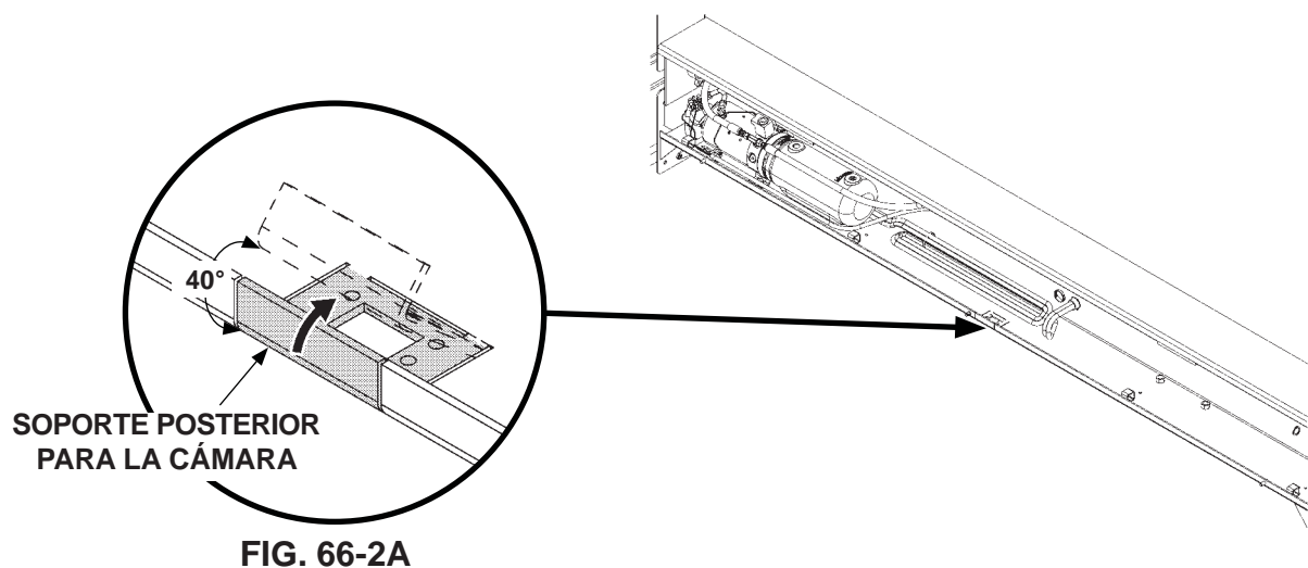
AJUSTAR EL SOPORTE DE LA CÁMARA FIG. 66-2
