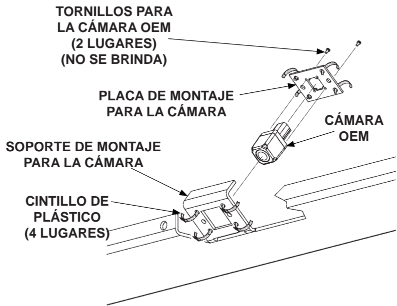
ACOPLAR LA CÁMARA A LA PLACA DE MONTAJE Y AL SOPORTE DE MONTAJE FIG. 67-2
