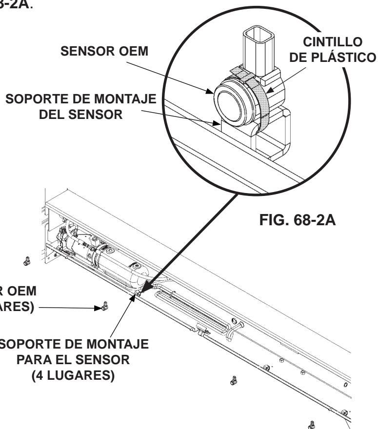
INSTALAR SENSORES (SI ESTÁN EQUIPADOS) FIG. 68-2
