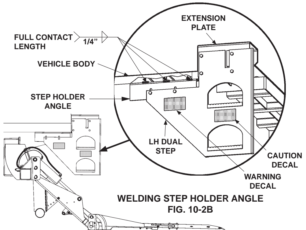
LH DUAL STEP SHOWN FIG. 10-2A
