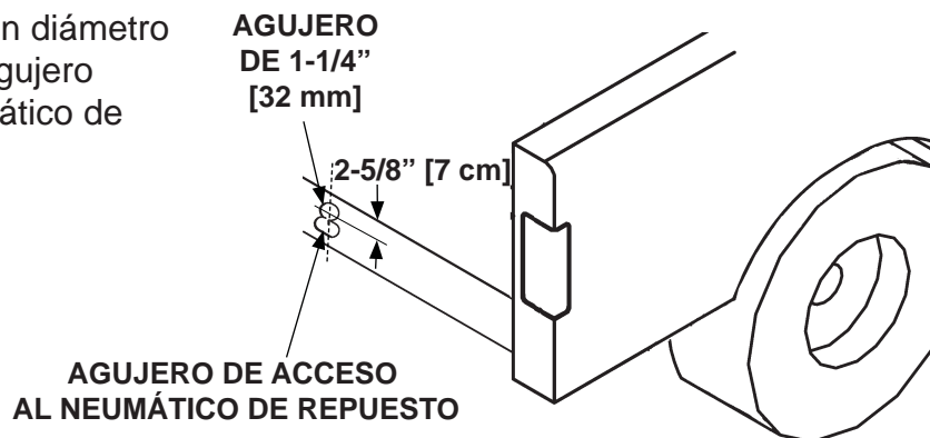
PERFORAR PARA EL MECANISMO DE MANIVELA EN NEUMÁTICO DE REPUESTO FIG. 38-2
