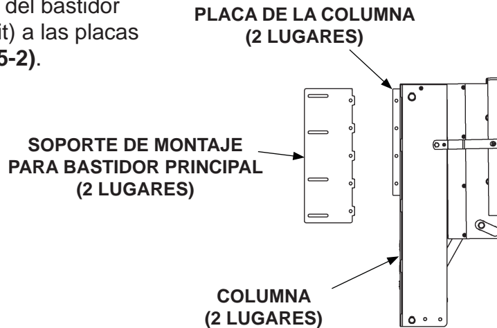
SE MUESTRA ELEVADOR C2 CON SOPORTES PARA ATORNILLAR EN EL BASTIDOR PRINCIPAL FIG. 35-1
