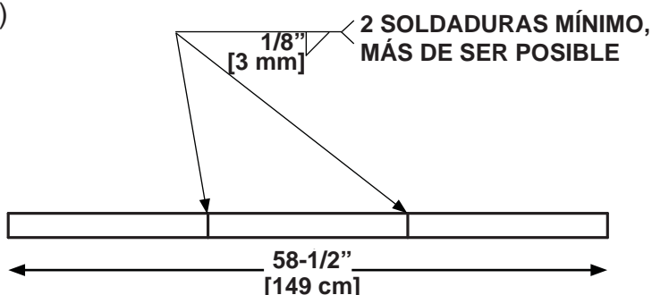
POSICIÓN Y SOLDADURAS PARA TIRA DE RELLENO FIG. 39-1
