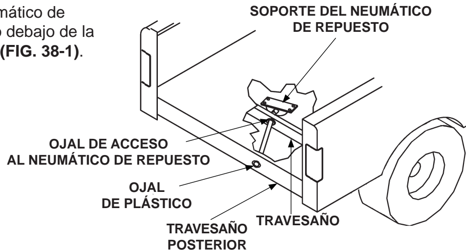
RETIRAR OJALES DE LOS TRAVESAÑOS DEL BASTIDOR FIG. 38-1
