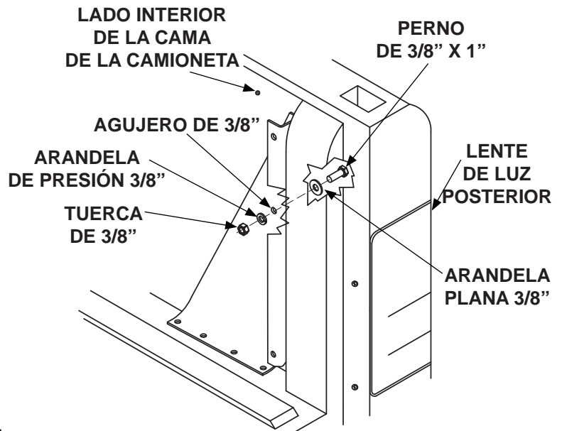
AJUSTAR SOPORTE A LA CAMA DE LA CAMIONETA (SE MUESTRA LADO DERECHO) FIG. 41-1
