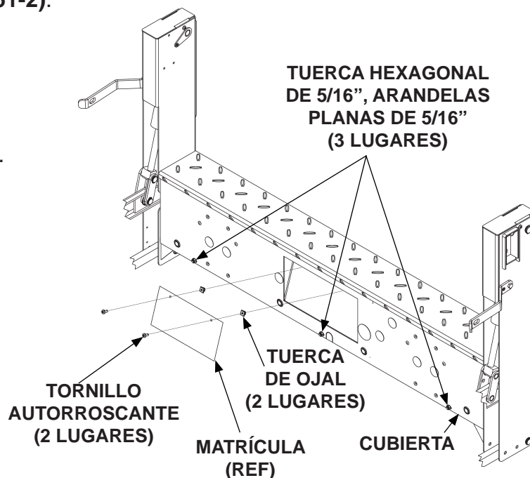
INSTALAR CUBIERTA Y MATRÍCULA (SE MUESTRA ELEVADOR C2) FIG. 51-2
