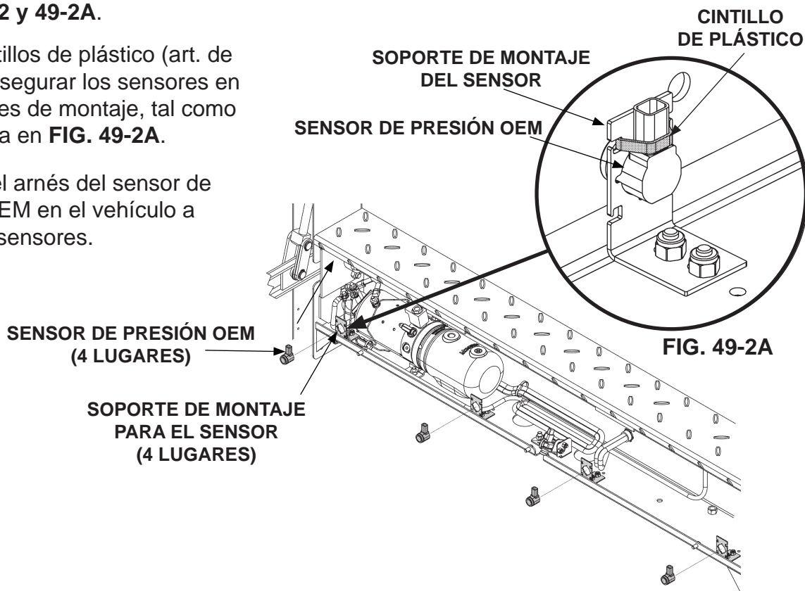
INSTALAR LOS SENSORES (SI SE EQUIPA) FIG. 49-2
