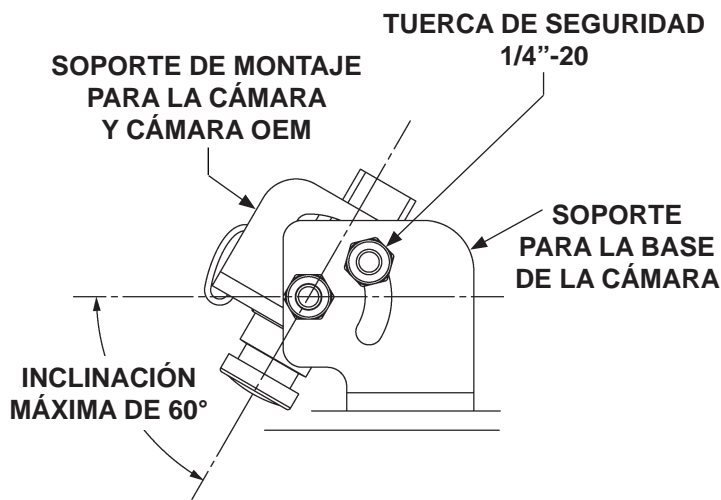
AJUSTAR EL ÁNGULO DE LA CÁMARA FIG. 49-1
