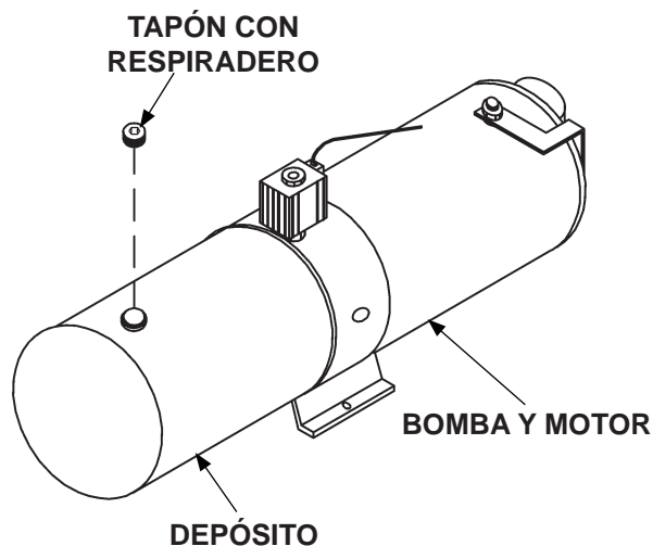
INSTALAR TAPÓN DE VENTILACIÓN EN EL DEPÓSITO DE LA BOMBA FIG. 51-1
