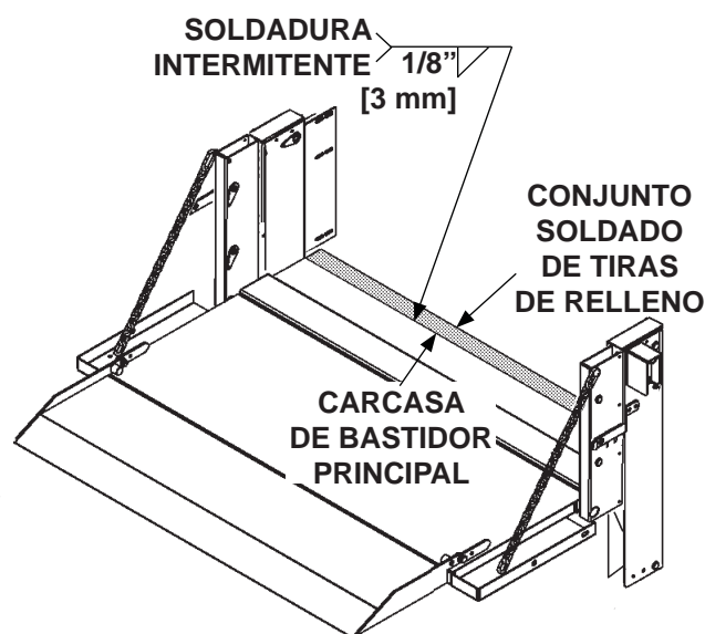
COLOCAR Y SOLDAR TIRA DE RELLENO FIG. 39-2
