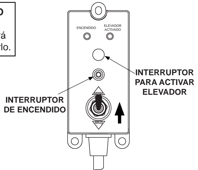
VERIFICAR LA OPERACIÓN DEL INTERRUPTOR Y ELEVAR LA PLATAFORMA FIG. 53-1
