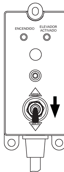
UTILIZAR INTERRUPTOR PARA DESCENDER EL ELEVADOR FIG. 42-1
