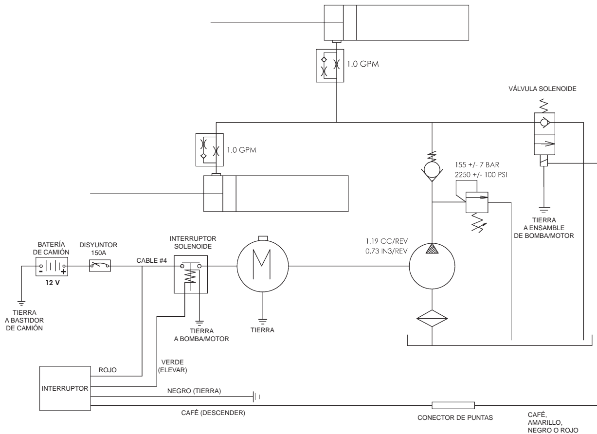
DIAGRAMA DE SISTEMAS ELÉCTRICOS E HIDRÁULICOS PARA ELEVADOR C2 FIG. 45-1
