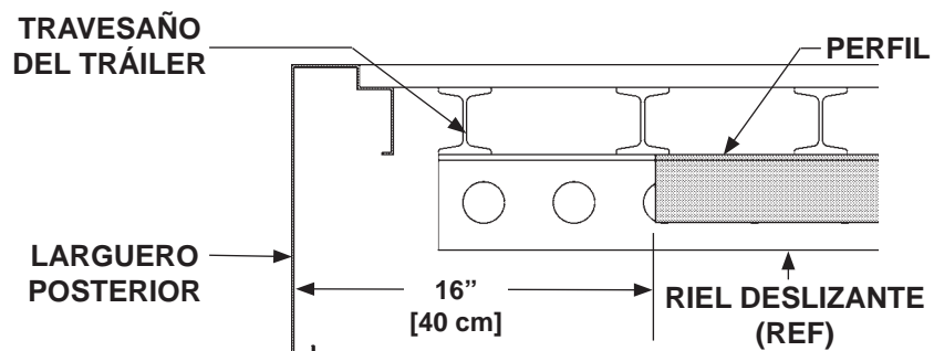
POSICIONAR PERFILES EN LOS TRAVESAÑOS DEL TRÁILER - VISTA LATERAL FIG. 12-3
