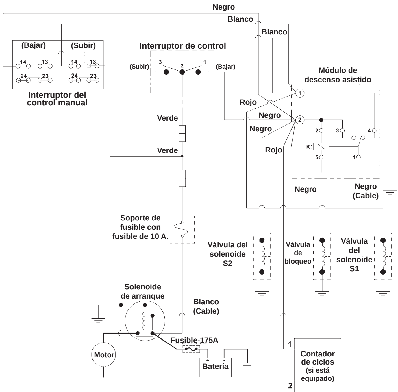
ESQUEMA ELÉCTRICO (DESCENSO ASISTIDO) CON CONTROL MANUAL FIG. 14-1
