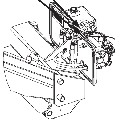
REEMPLAZAR EL OJAL FIG. 19-1
