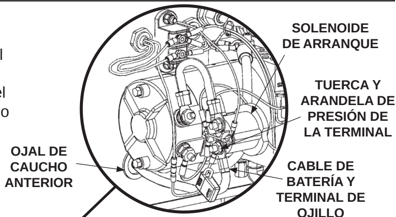
OJAL DE CAUCHO ANTERIOR FIG. 19-1A
