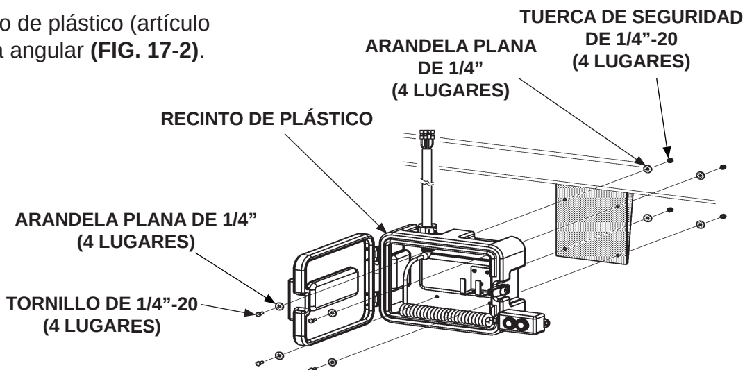
ATORNILLAR RECINTO A LA PLACA ANGULAR FIG. 17-2
