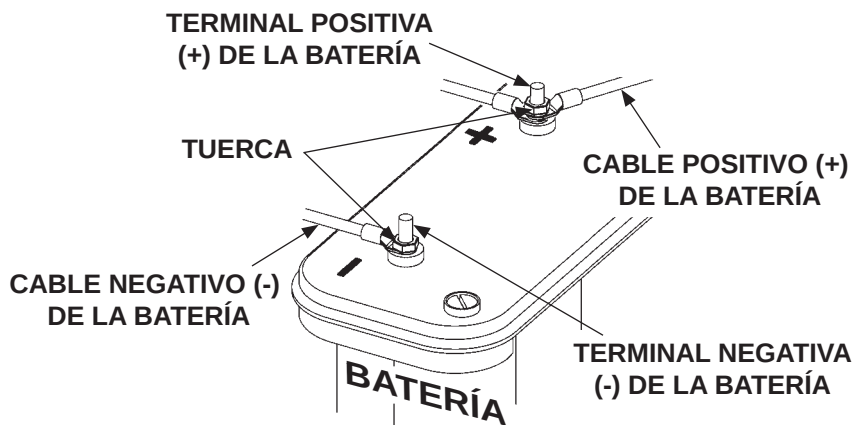
CABLES DE LA BATERÍA RECONECTADOS FIG. 21-2
