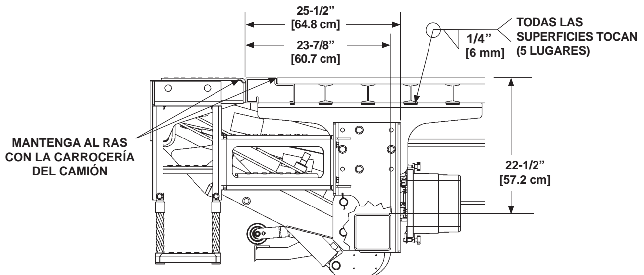
SOLDAR EL ELEVADOR AL CHASIS DEL ELEVADOR (SE MUESTRA EL LADO DERECHO)
