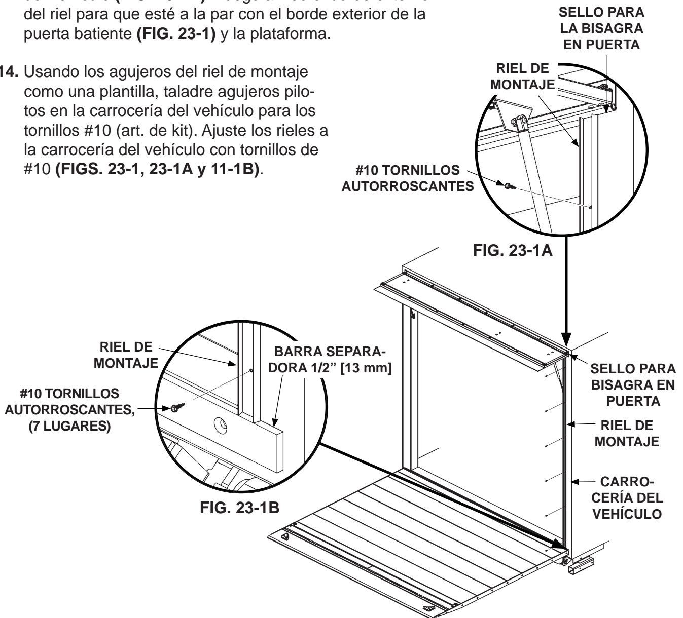
INSTALAR RIELES DE MONTAJE FIG. 23-1
