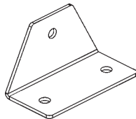
SOPORTE EN ÁNGULO, AGUJEROS 3 X 5/16" DIÁMETRO N/P 212000-P1 CANT. 2
