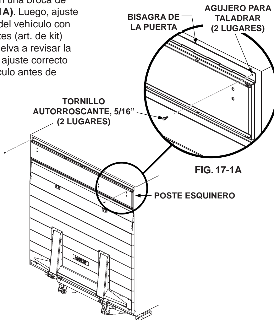
ATORNILLAR LA PUERTA BATIENTE FIG. 17-1
