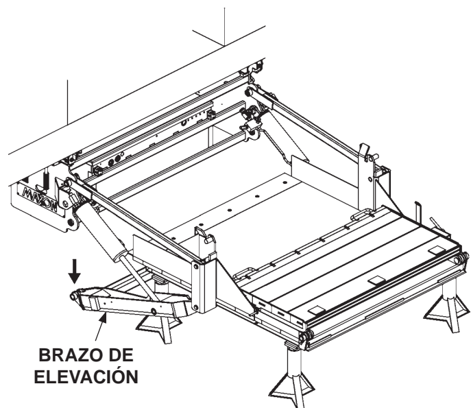
DESCENDER EL BRAZO DE ELEVACIÓN EN EL BASTIDOR (SE MUESTRA LADO IZQ.) FIG. 11-2
