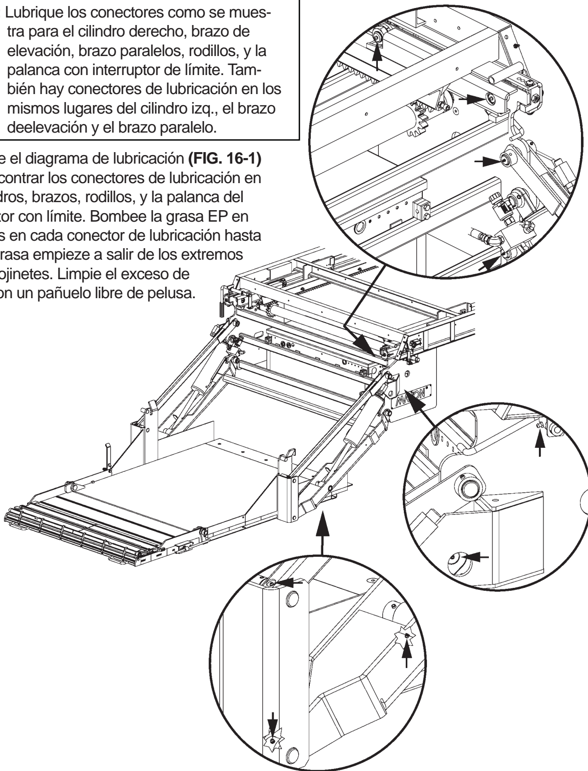
DIAGRAMA DE LUBRICACIÓN RA FIG. 16-1
