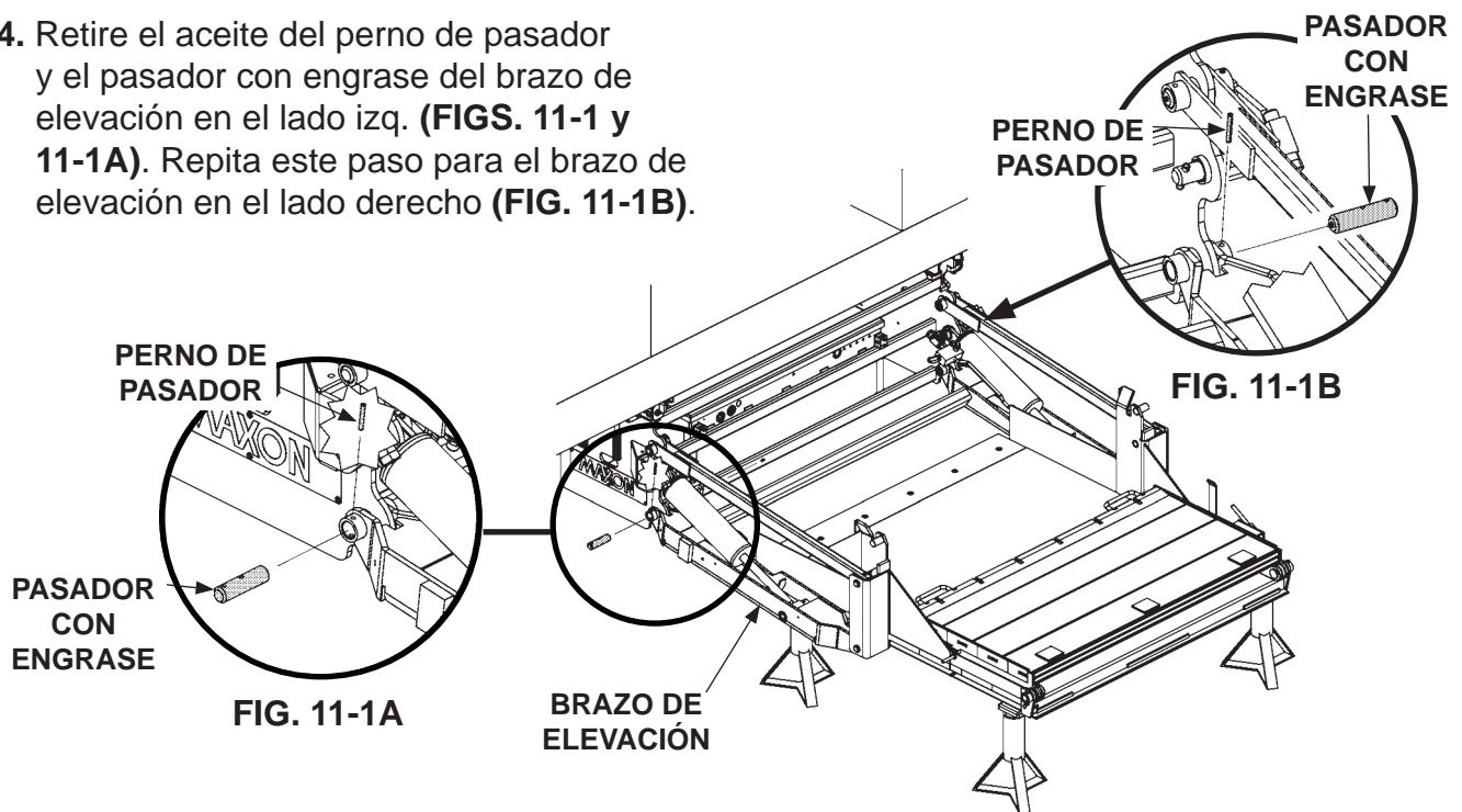
RETIRAR EL BRAZO DE ELEVACIÓN EN EL PASADOR CON ENGRASE (SE MUESTRA LADO IZQ.) FIG. 11-1
