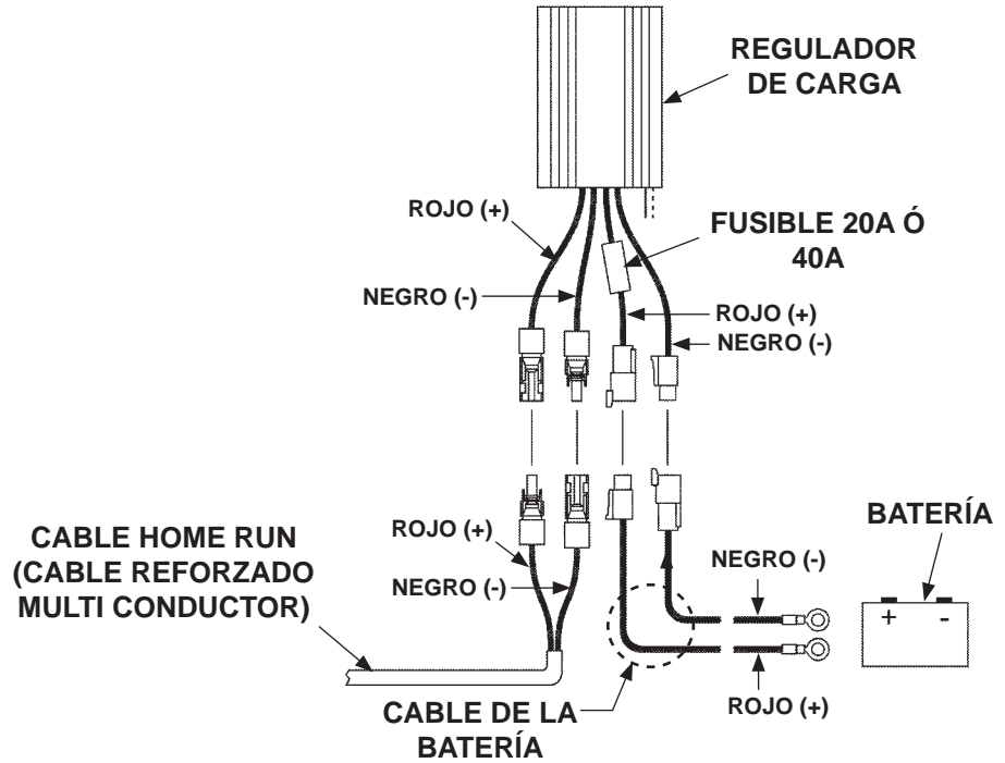
CONECTAR EL HOME RUN CABLE (CABLE REFORZADO MULTI CONDUCTOR) Y LOS CABLES DE LA BATERÍA AL REGULADOR DE CARGA FIG. 27-1
