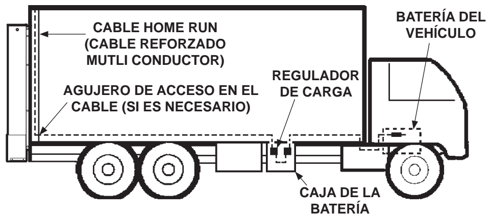
INSTALAR UN CABLE HOME RUN A LA CAJA DE LA BATERIA FIG. 26-2
