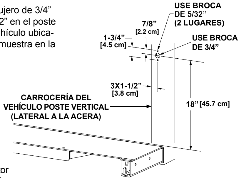
PERFORAR AGUJEROS DE MONTAJE FIG. 42-1
