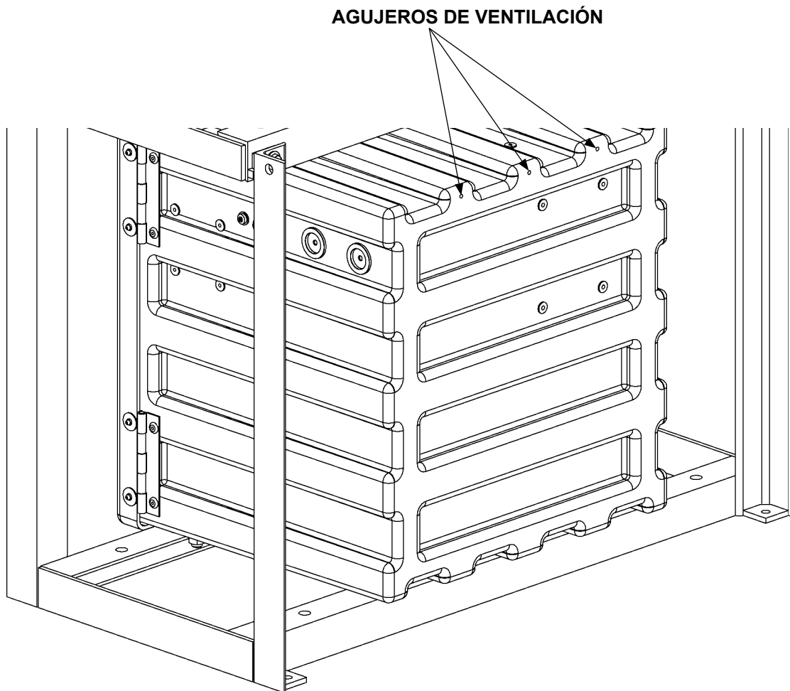
ENSAMBLE DE LA CAJA DE BATERÍA (SE MUESTRA VISTA POSTERIOR) FIG. 34-1
