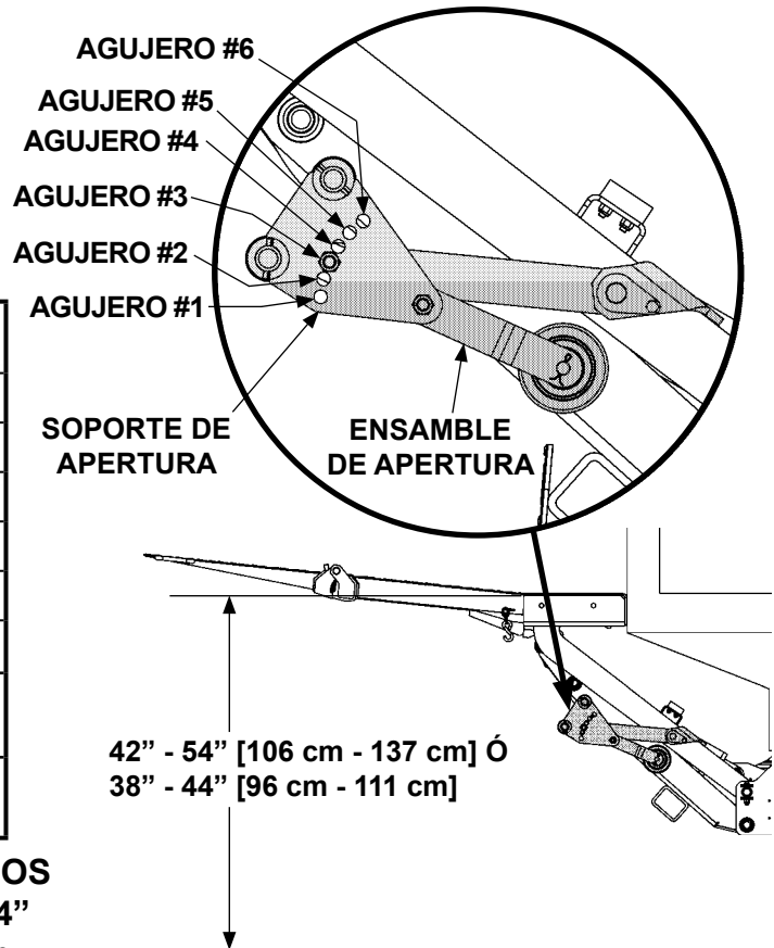
AJUSTANDO EL BRAZO DE APERTURA PARA CAMA BAJA DE 38" - 44" [96 cm - 111 cm] O CAMA ALTA DE 42" - 54" [106 cm - 137 cm] FIG. 52-2
