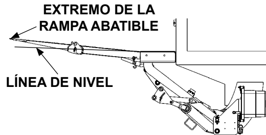
EXTREMO DE LA RAMPA ABATIBLE LÍNEA DE NIVEL EL BORDE DE LA PLATAFORMA ARRIBA DEL NIVEL DE CAMA FIG. 54-2
