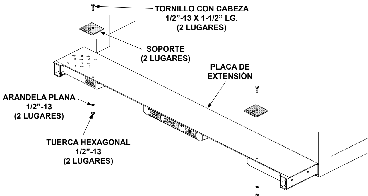
ATORNILLAR LOS SOPORTES DE INSTALACIÓN FIG. 21-2
