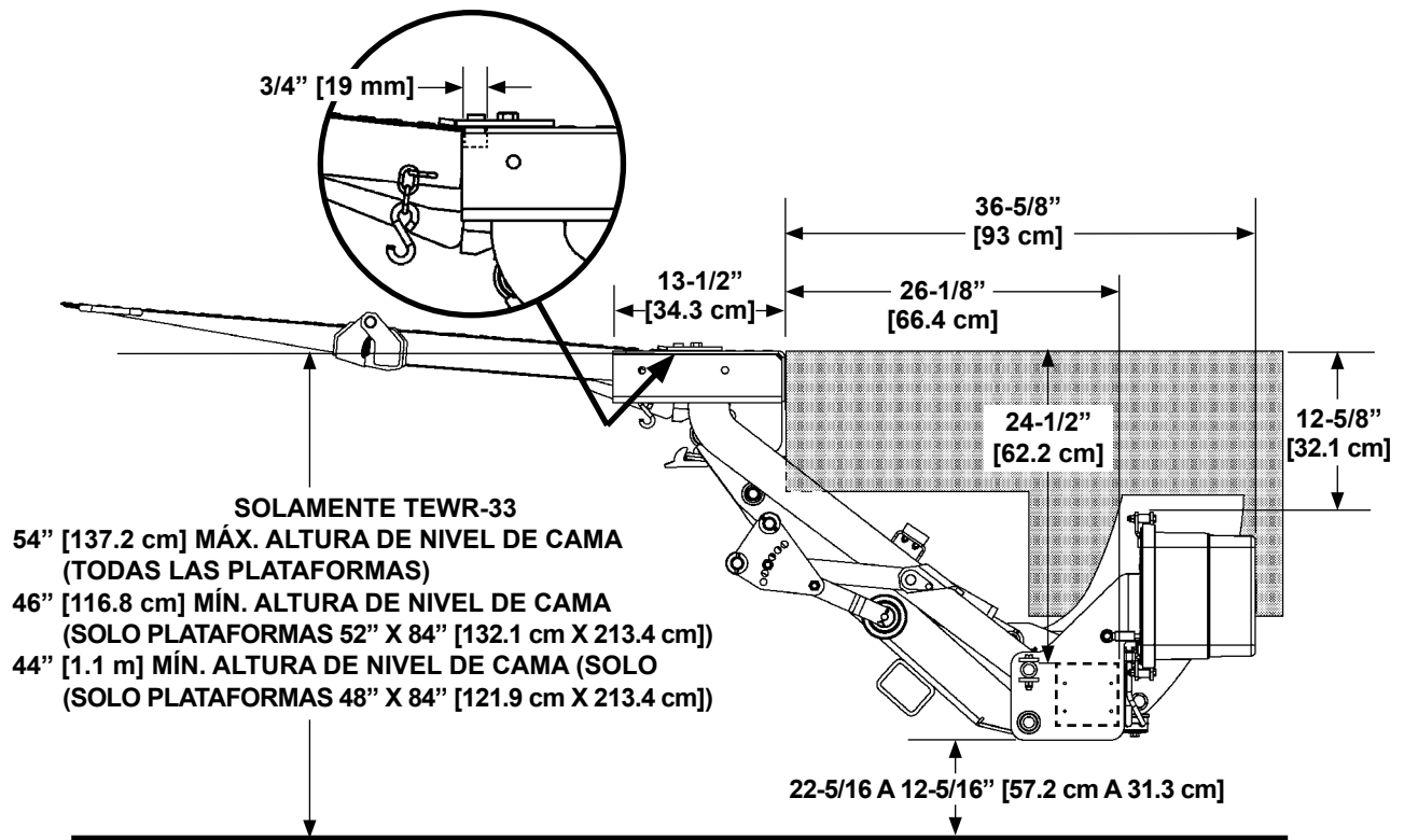
DIMENSIONES DE TEWR-33 RAMPA PARA CAMINAR FIG. 11-2
