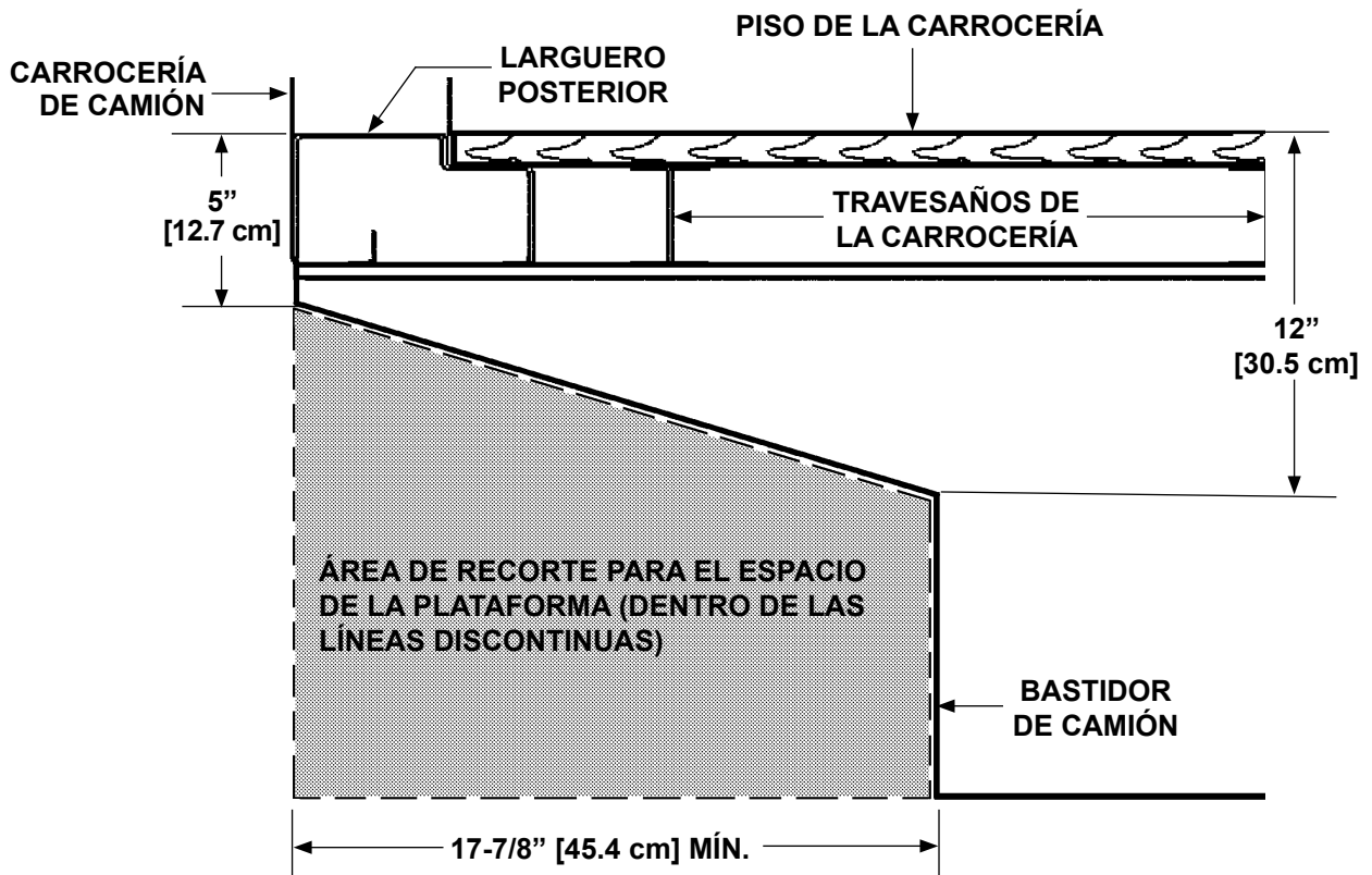
RECORTE DEL BASTIDOR DEL VEHÍCULO PARA EL ESPACIO DE LA PLATAFORMA (ALTURA DE CAMA 54" A 42" [137.2 cm A 106.7 cm]) FIG. 13-1
