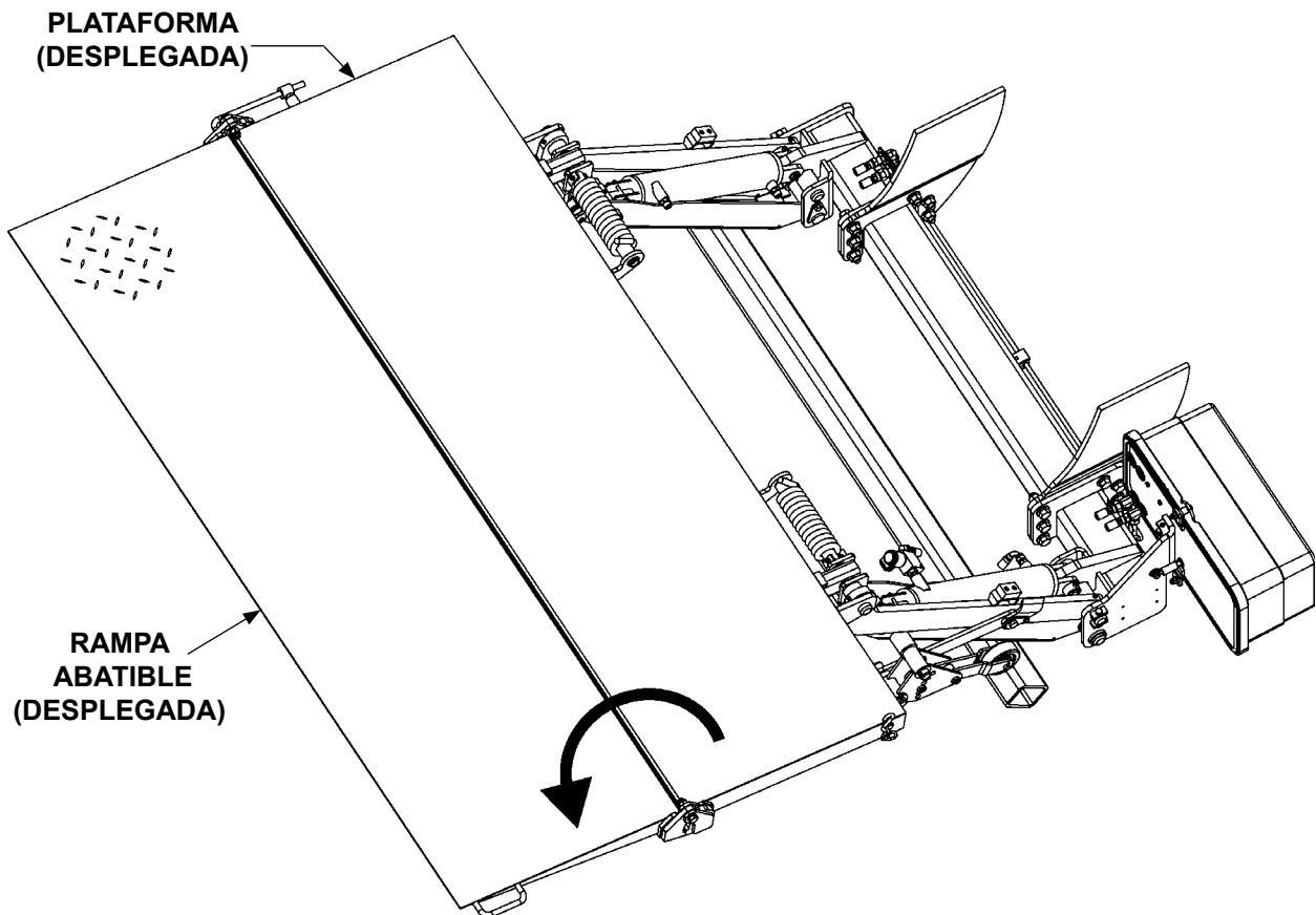
PLATAFORMA Y RAMPA ABATIBLE DESPLÉGADAS FIG. 23-2
