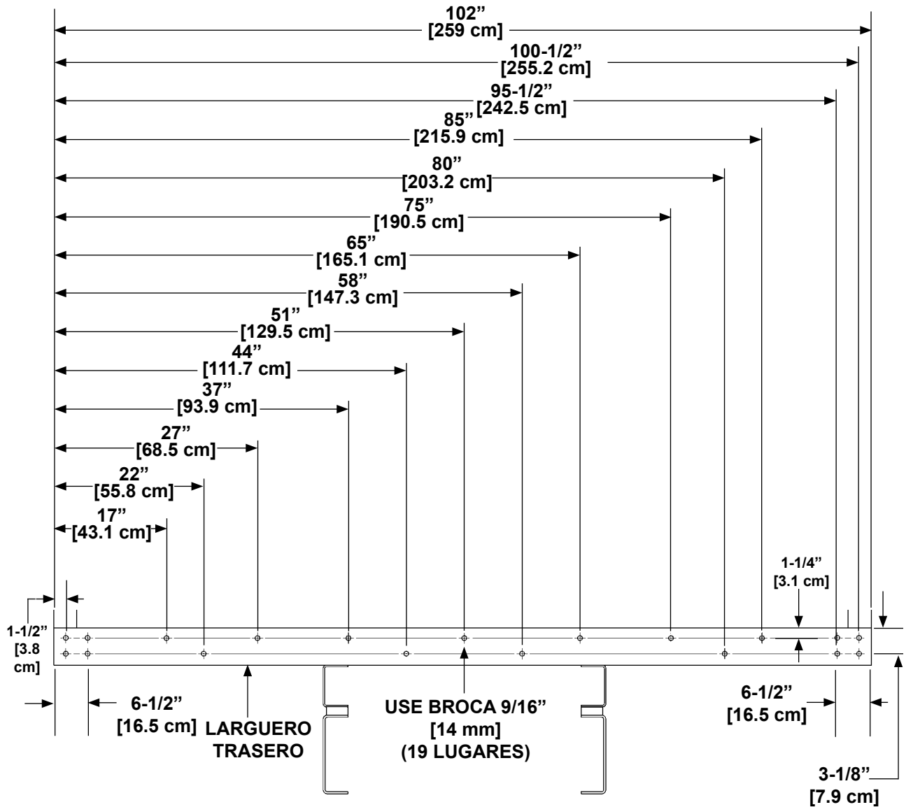
LARGUERO POSTERIOR - UBICACIÓN DE AGUJEROS PARA VEHÍCULOS DE 102" [259 cm] DE ANCHO FIG. 18-1
