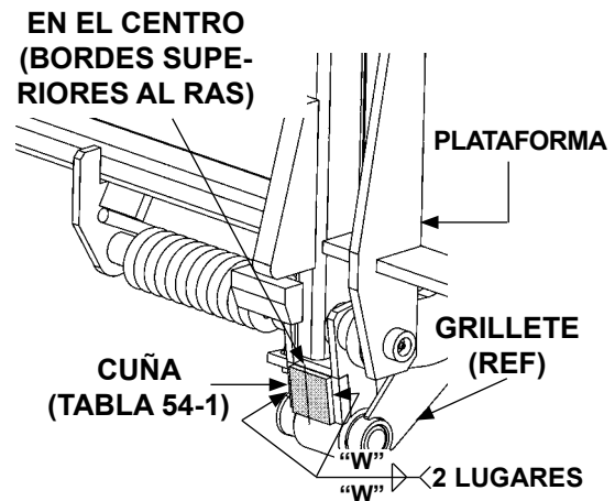
EN EL CENTRO (BORDES SUPERIORES AL RAS) SOLDAR CUÑAS (LATERAL A LA ACERA) FIG. 54-4
