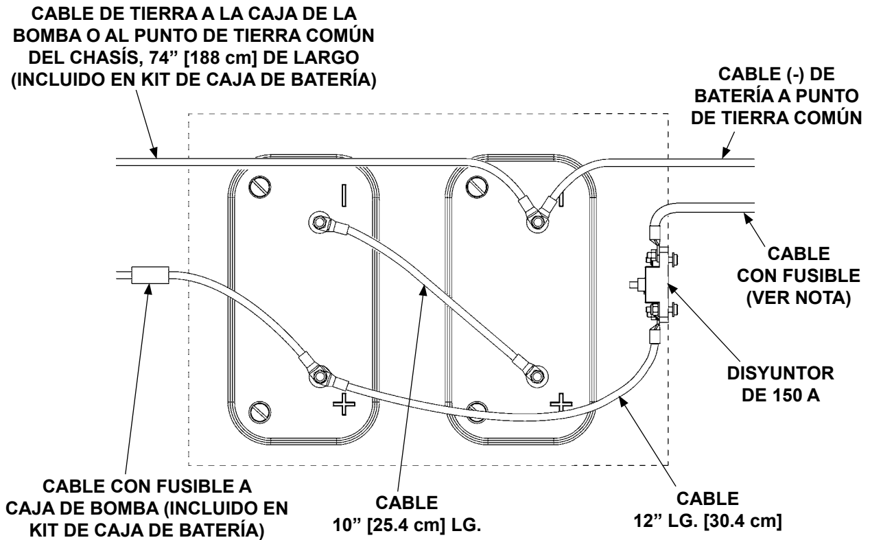
CONEXIONES DE BATERÍA DE 12 V PARA ALIMENTACIÓN DE 24 V FIG. 33-1
