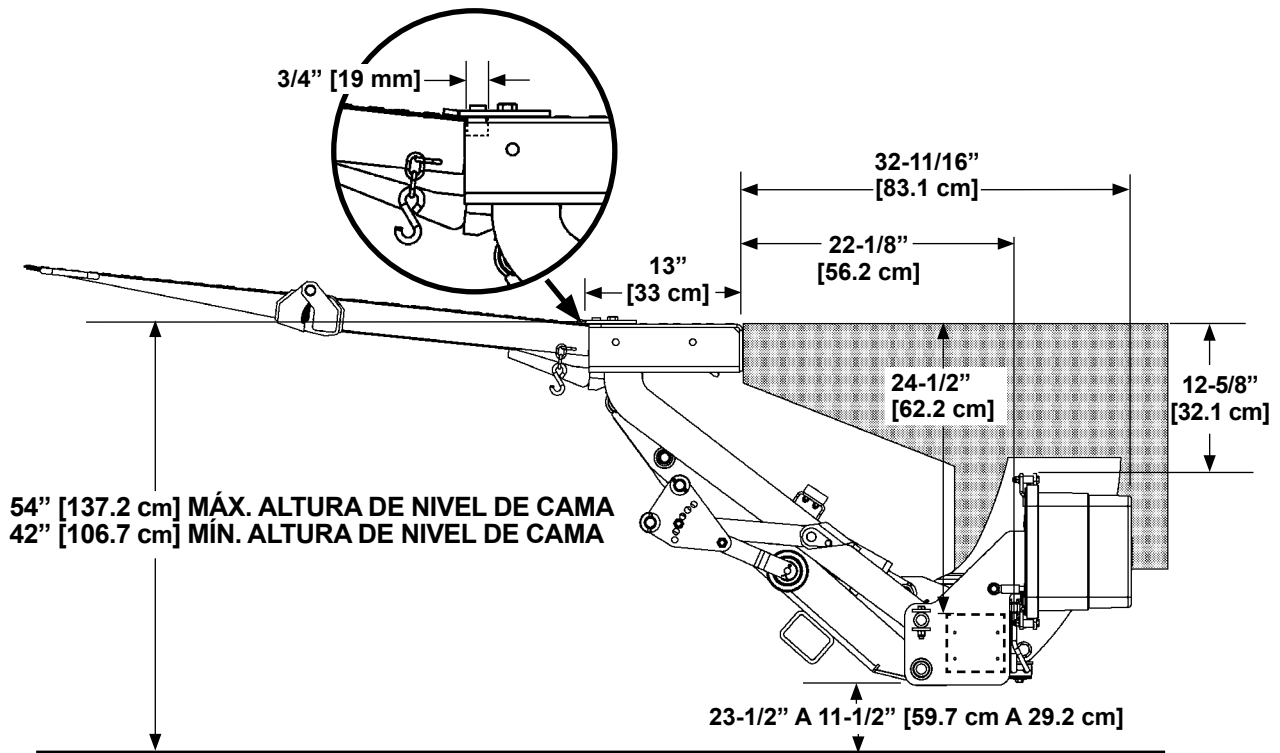
DIMENSIONES TE-33 ALTURA DE CAMA FIG. 10-1
