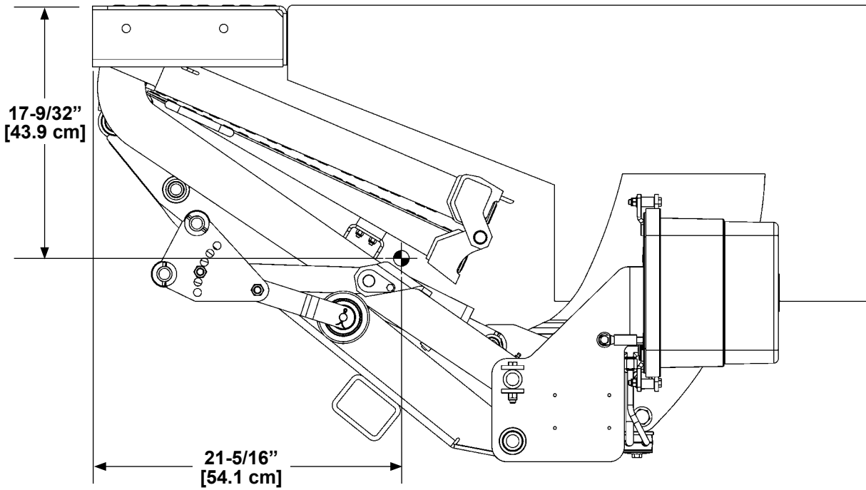
CENTRO DE MASA PARA TE-33 (POSICIÓN DE GUARDADO) FIG. 16-1
