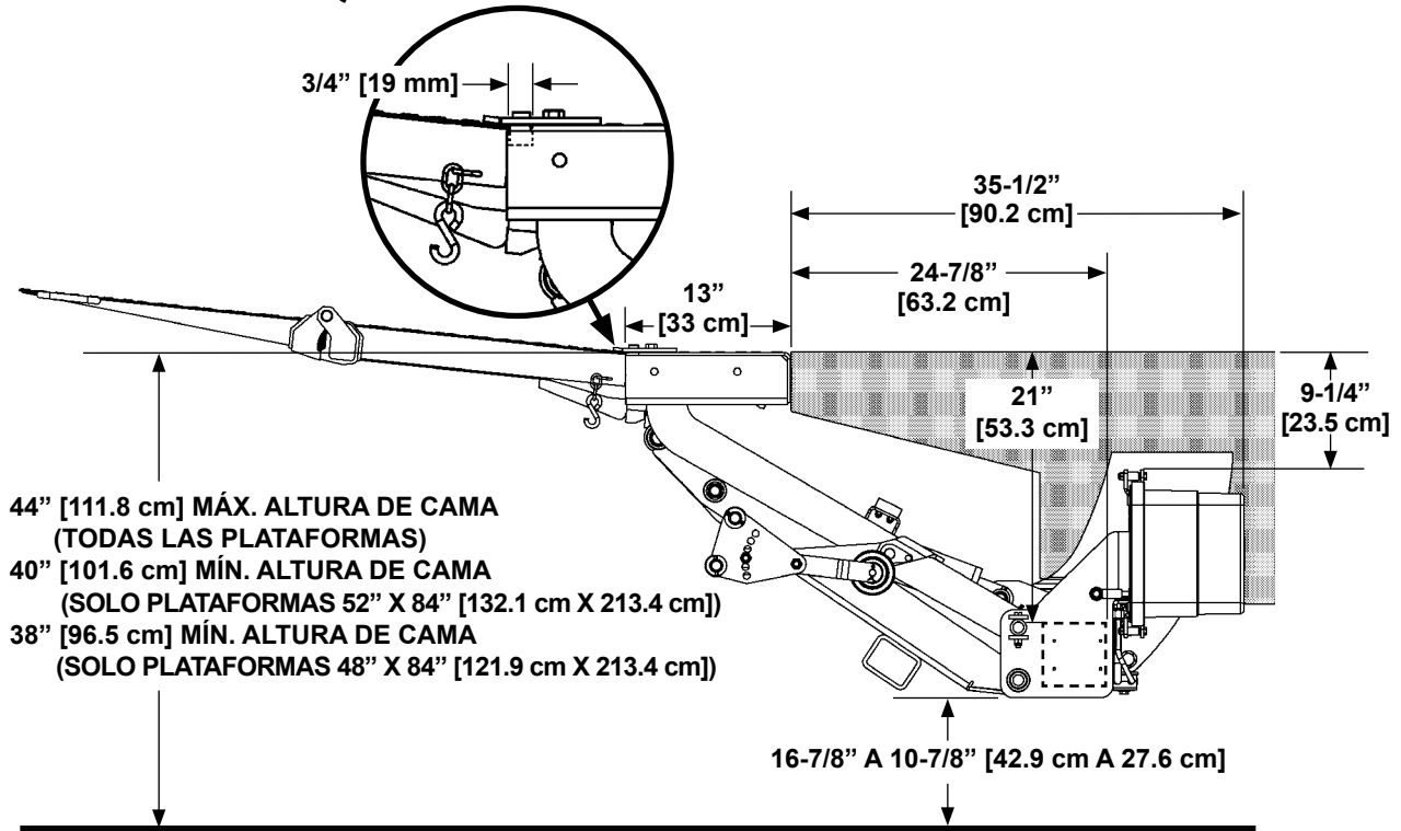
DIMENSIONES TE-33 ALTURA DE CAMA FIG. 11-1
