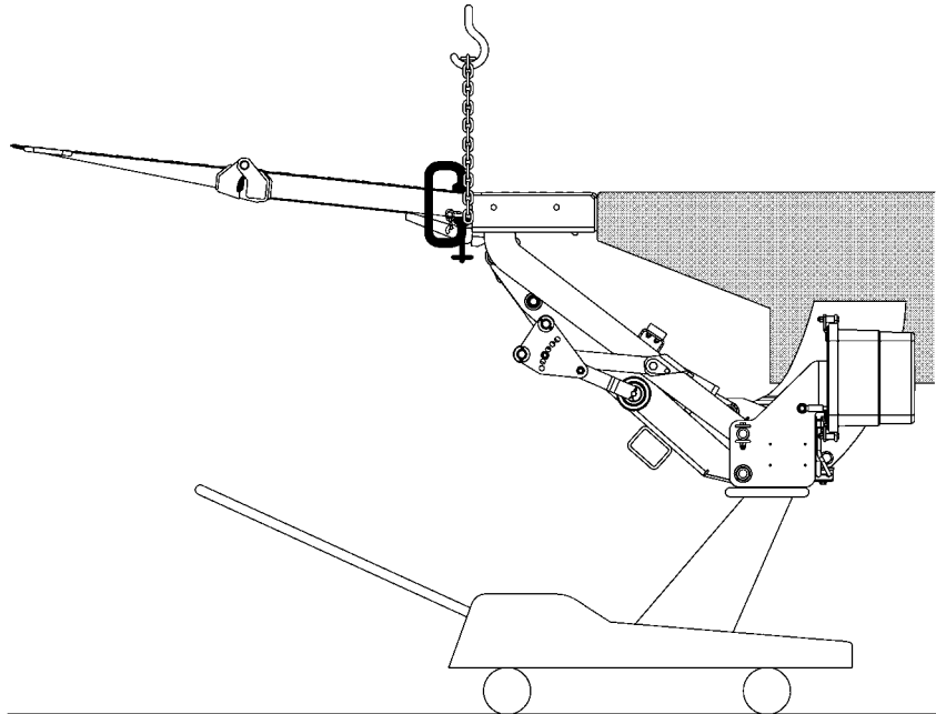
MANERA CORRECTA DE ENGANCHAR LA GRÚA AL ELEVADOR FIG. 24-1
