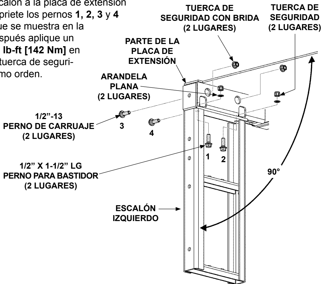
ATORNILLAR EL ESCALÓN A LA PLACA DE EXTENSIÓN (SE MUESTRA ESCALÓN DOBLE IZQUIERDO) FIG. 58-1
