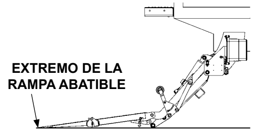
EXTREMO DE LA RAMPA ABATIBLE LA PLATAFORMA Y GRILLETES TOCAN EL SUELO FIG. 54-1
