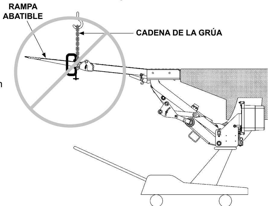
MANERA INCORRECTA DE ENGANCHAR EL ELEVADOR FIG. 24-2
