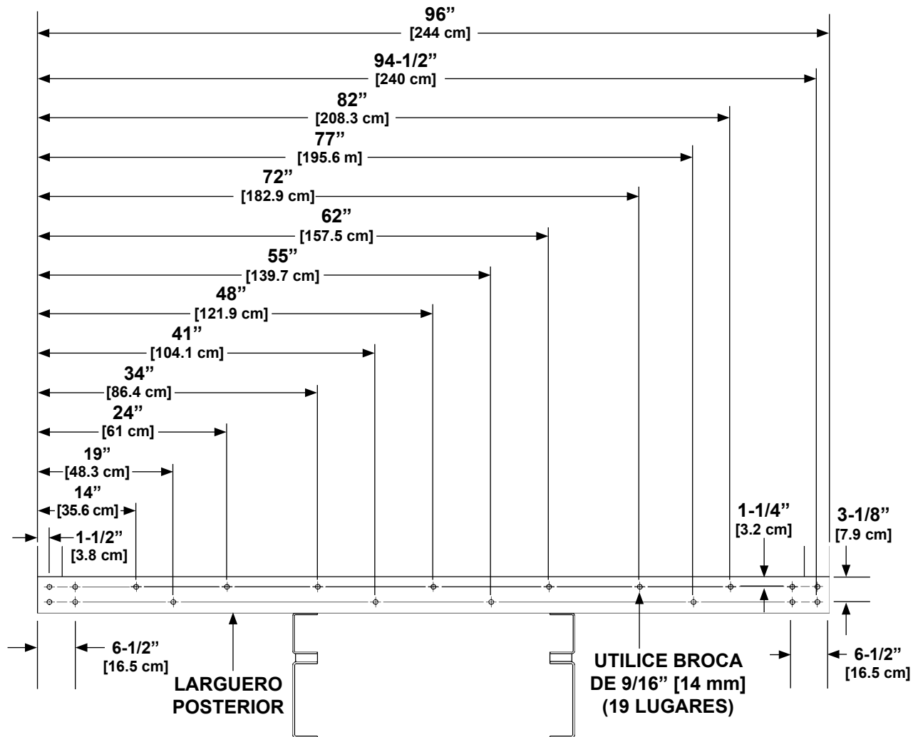
LARGUERO POSTERIOR - UBICACIÓN DE AGUJEROS PARA VEHÍCULOS DE 96" [244 cm] DE ANCHO FIG. 17-1
