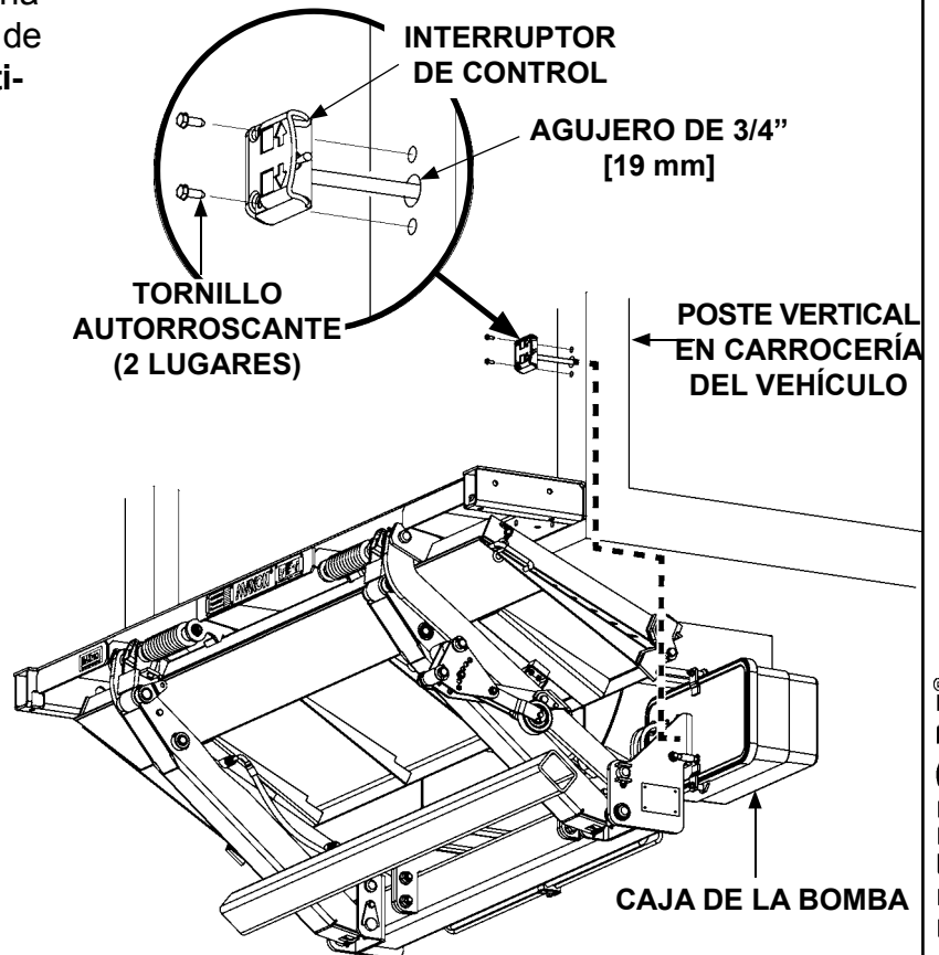
GUÍE EL CABLEADO DEL INTERRUPTOR DE CONTROL FIG. 42-2
