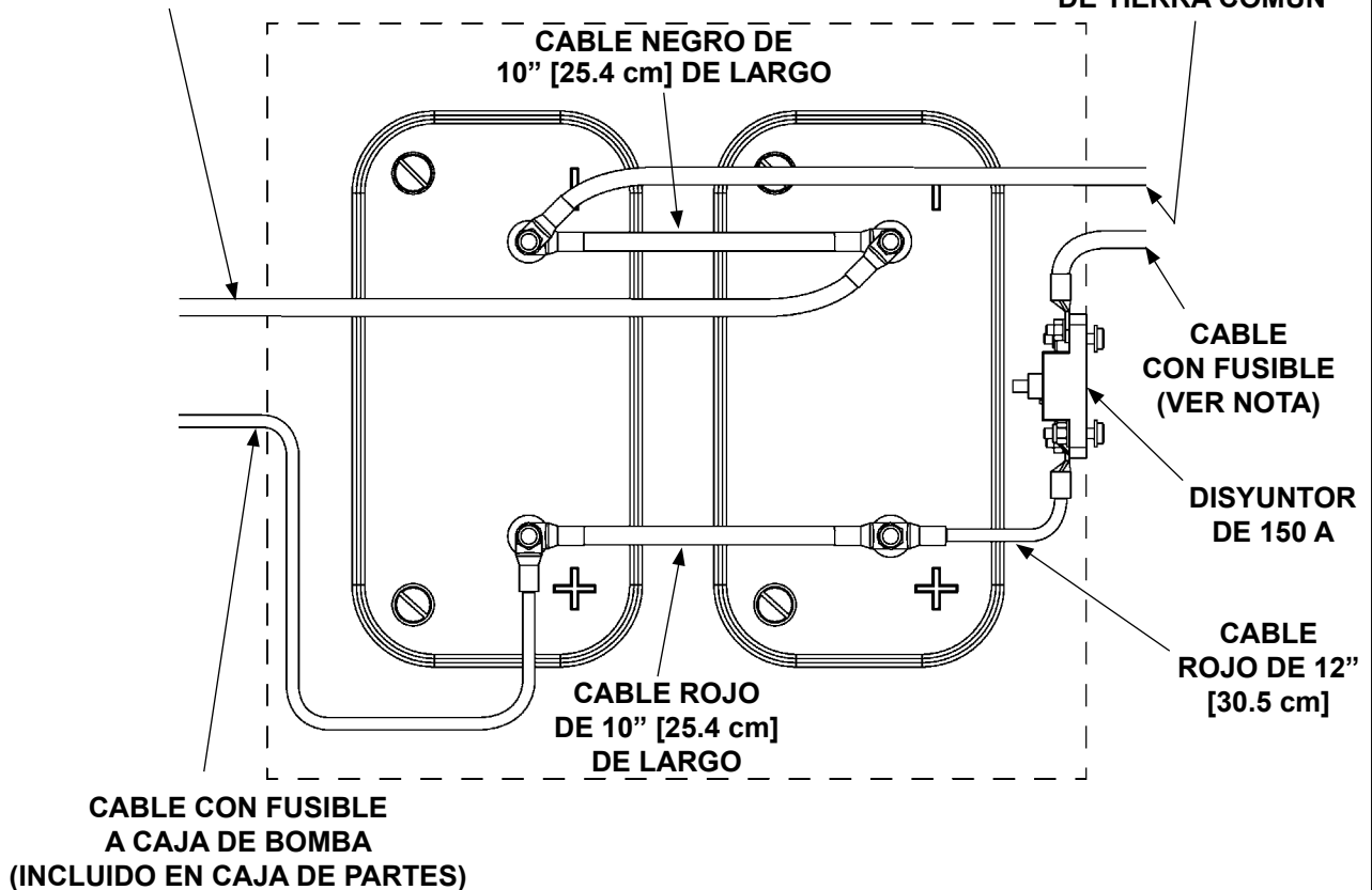
CONEXIONES DE BATERÍA DE 12 V PARA ALIMENTACIÓN DE 12 V FIG. 32-1
