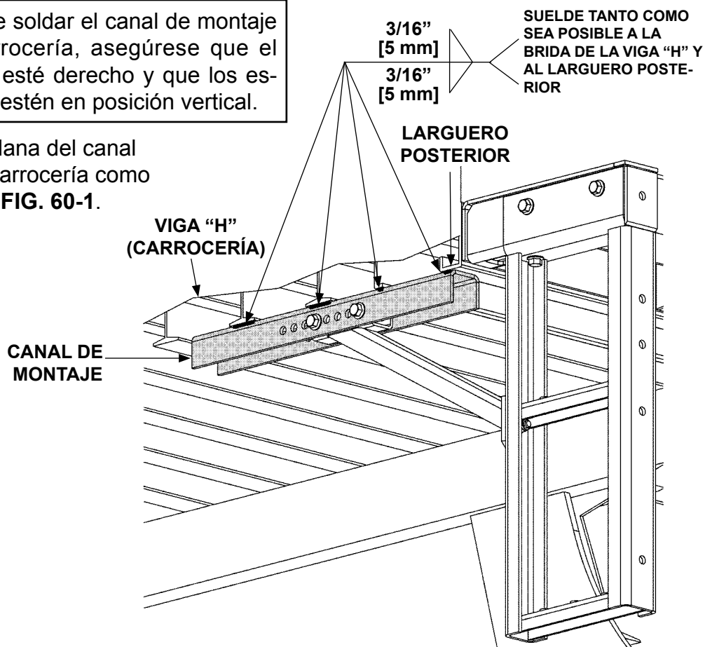
SOLDAR LA PARTE PLANA DEL CANAL DE MONTAJE A LA CARROCERÍA (SE MUESTRA ESCALÓN DOBLE IZQUIERDO) FIG. 60-1
