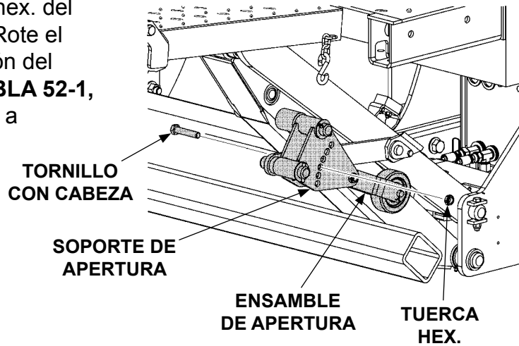
RETIRAR EL PERNO DEL SOPORTE DE APERTURA FIG. 52-1
