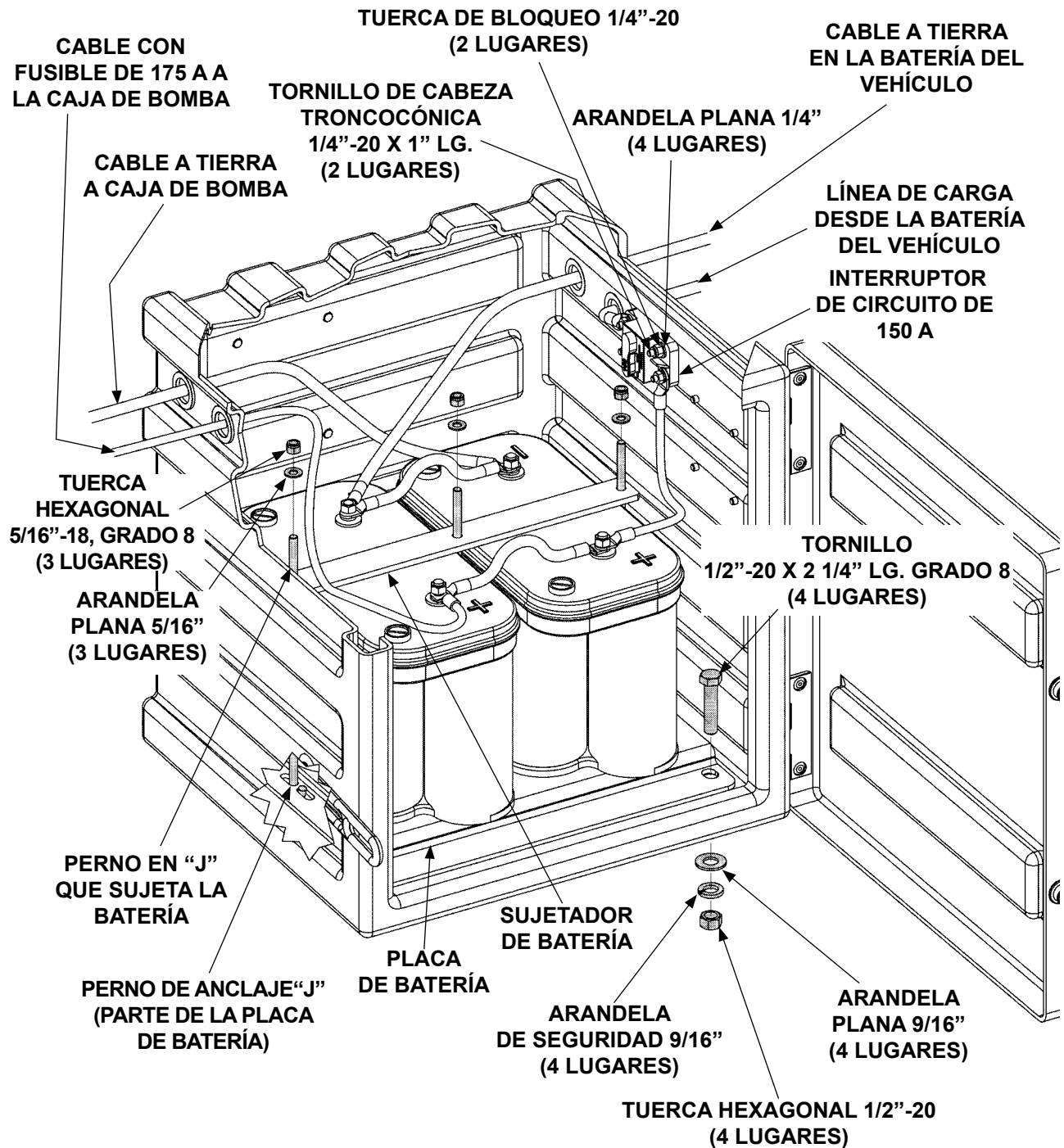
ENSAMBLE DE LA CAJA DE BATERÍA (SE MUESTRAN CONEXIONES DE 12 V) FIG. 35-1
