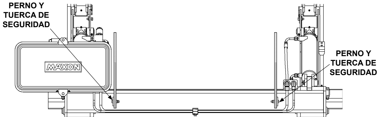
PLACAS DE MONTAJE PARA SOLDAR (PINTADAS), SE ATORNILLAN TEMPORALMENTE COMO SE MUESTRAN FIG. 23-1
