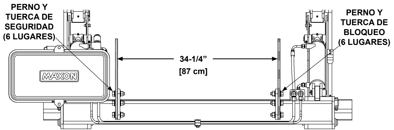
PLACAS DE MONTAJE PARA ATORNILLAR DE 34-1/4" [87 cm] FIG. 22-1
