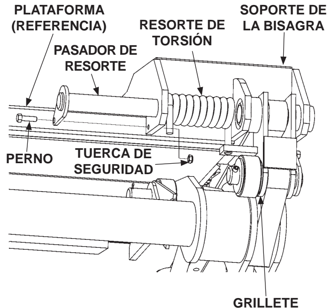
RETIRAR RESORTE Y PASADOR DE RESORTE FIG. 8-1
