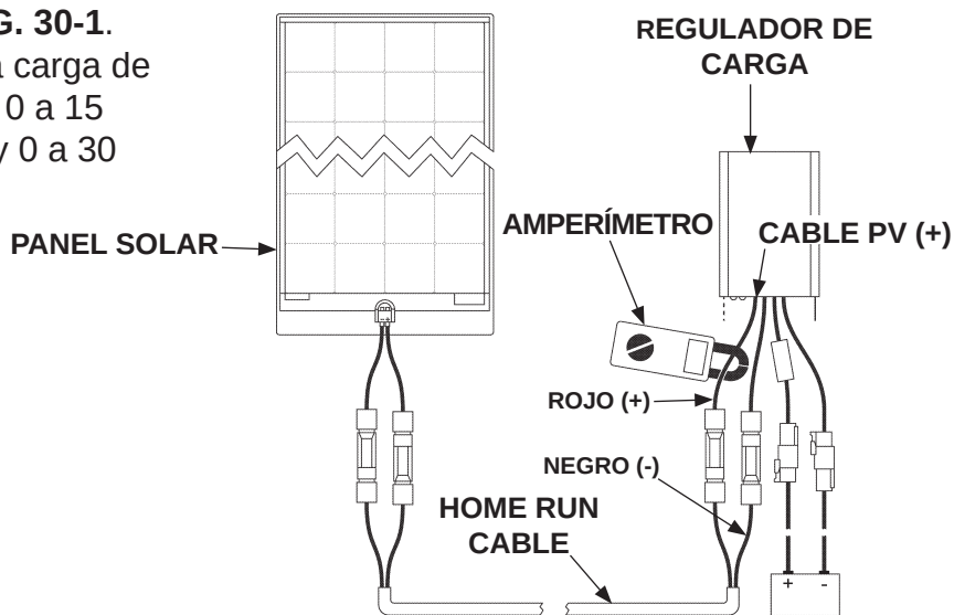
MEDIR LA CORRIENTE EN EL CABLE PV (+) FIG. 30-1
