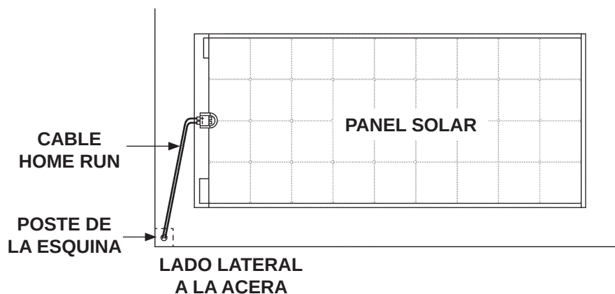
INSTALAR EL CABLE HOME RUN A TRAVÉS DEL POSTE EN LA ESQUINA FIG. 26-1
