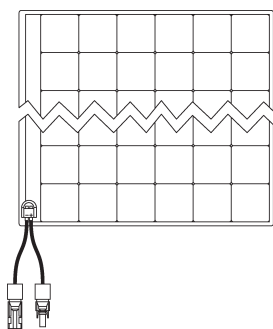
PANEL SOLAR 6 X 12 CON CABLES EN LA CAJA DE CONEXIONES, 360W N/P 211629-01 CANT. 1
