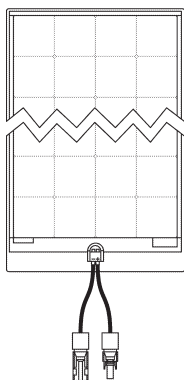
PANEL SOLAR 4 X 12 CON CABLES EN LA CAJA DE CONEXIONES, 240W N/P 211628-01 CANT. 1
