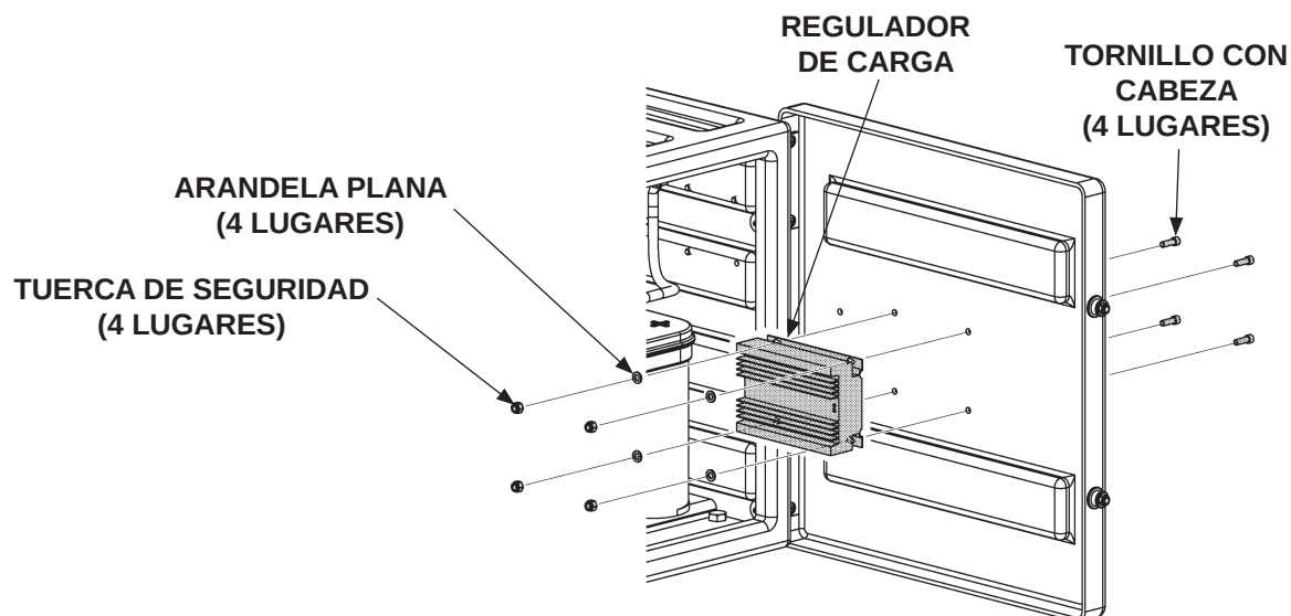
ATORNILLAR EL REGULADOR DE CARGA TS-30 FIG. 24-2
