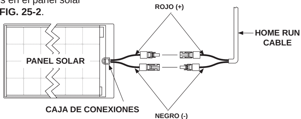
CONECTAR EL PANEL SOLAR AL CABLE HOME RUN FIG. 25-2
