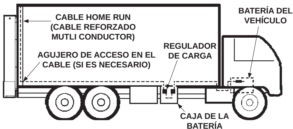
INSTALAR UN CABLE HOME RUN A LA CAJA DE LA BATERIA FIG. 26-2
