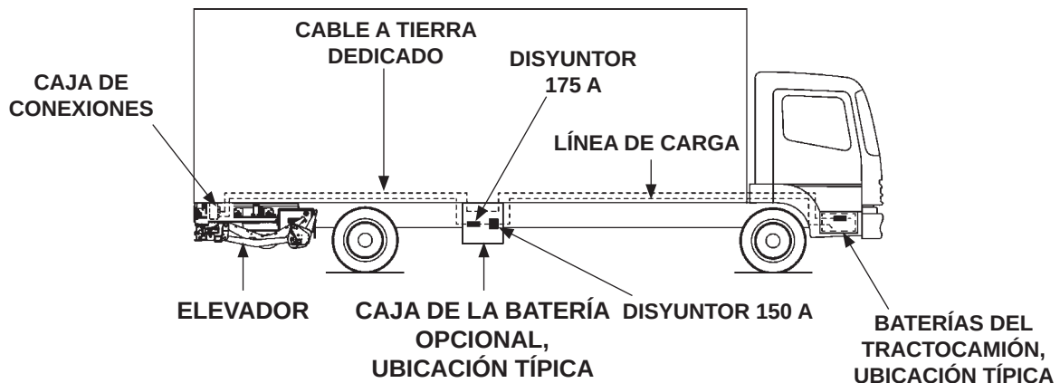
CAJA DE BATERÍA OPCIONAL INSTALADA EN TRACTOCAMIÓN (SE MUESTRA RA) FIG. 35-2
