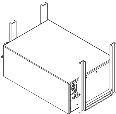
ENSAMBLE DE LA CAJA CON 4 BATERÍAS N/P 289690-11, 289690-12, 289690-13 CANT. 1
