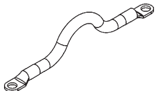
ENSAMBLE DEL CABLE ROJO, CALIBRE 2, 8" [20.3 cm] DE LARGO N/P 269308-10 CANT. 2
