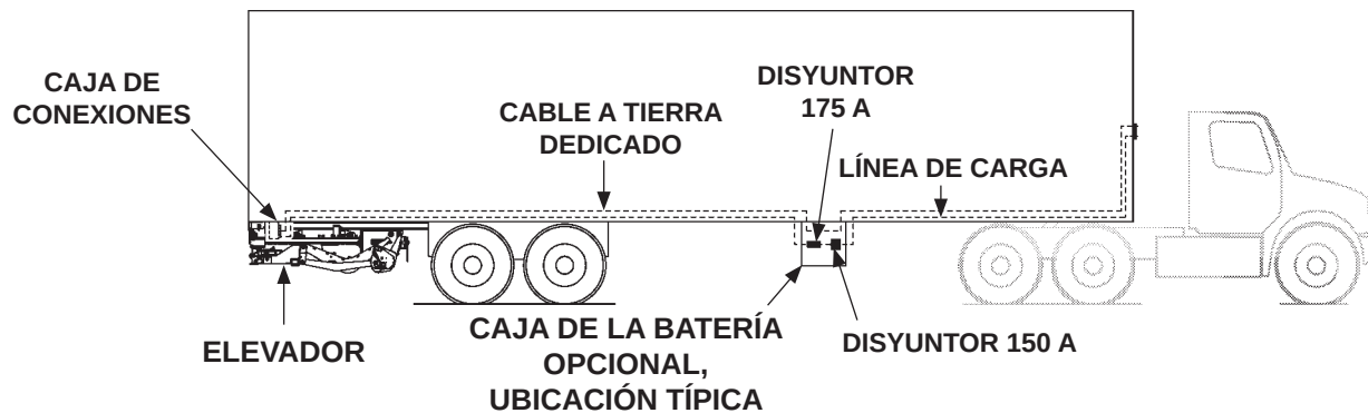
CAJA DE BATERÍA OPCIONAL INSTALADA EN TRÁILER (SE MUESTRA GPSLR) FIG. 35-1
