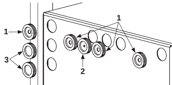
UBICACIONES DEL OJAL DE CAUCHO PARA EL KIT N/P 289690-02 FIG. 45-2
