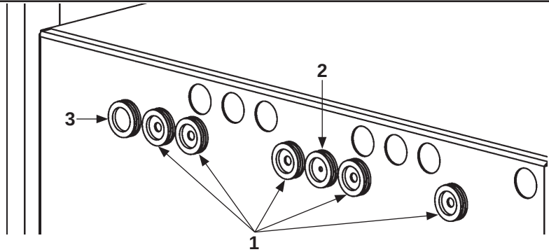
UBICACIONES DEL OJAL DE CAUCHO PARA EL KIT N/P 289690-11 FIG. 46-1
