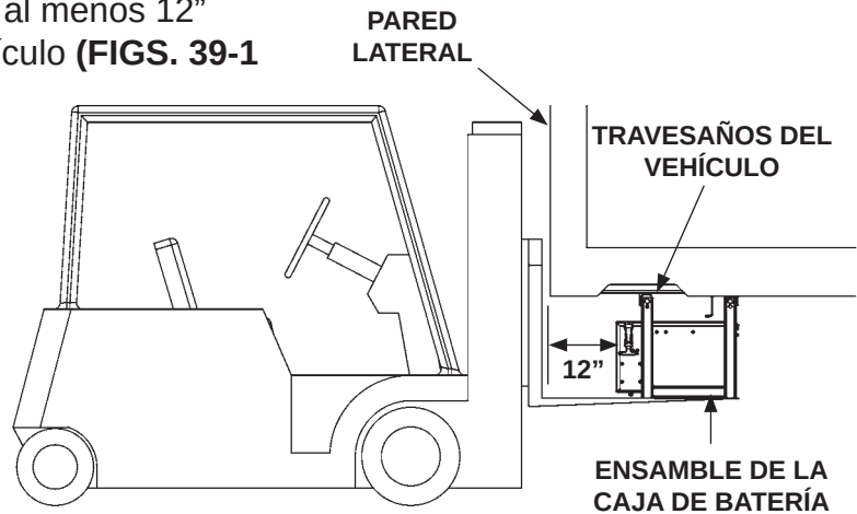
POSICIONAR ENSAMBLE DE LA CAJA DE BATERÍA FIG. 39-1
