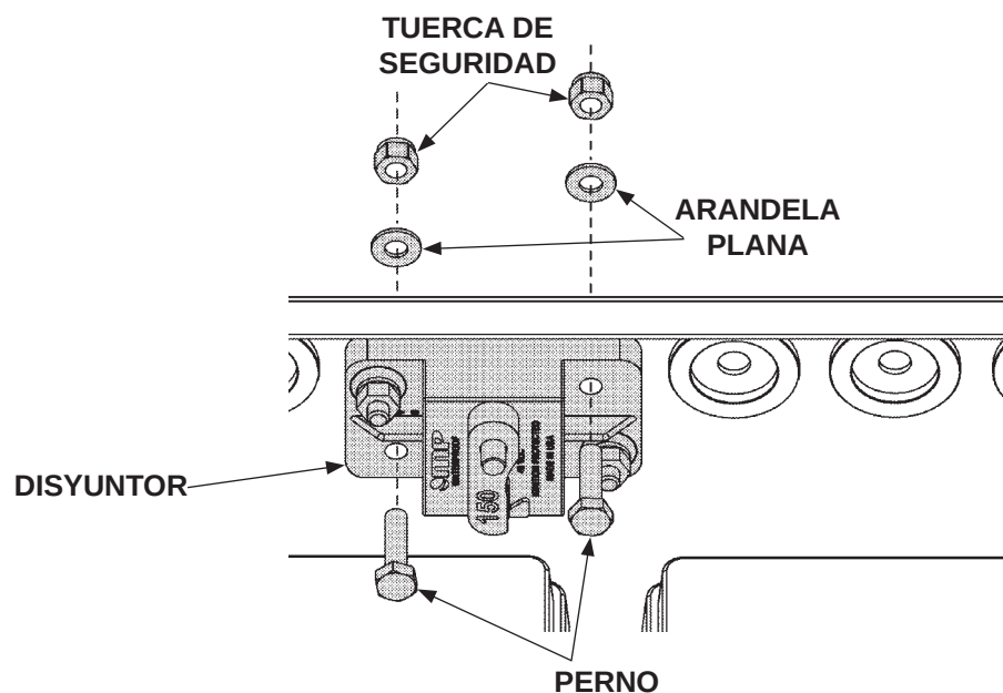
MONTAR EL DISYUNTOR (CAJA CON 4 BATERÍAS) FIG. 43-2
