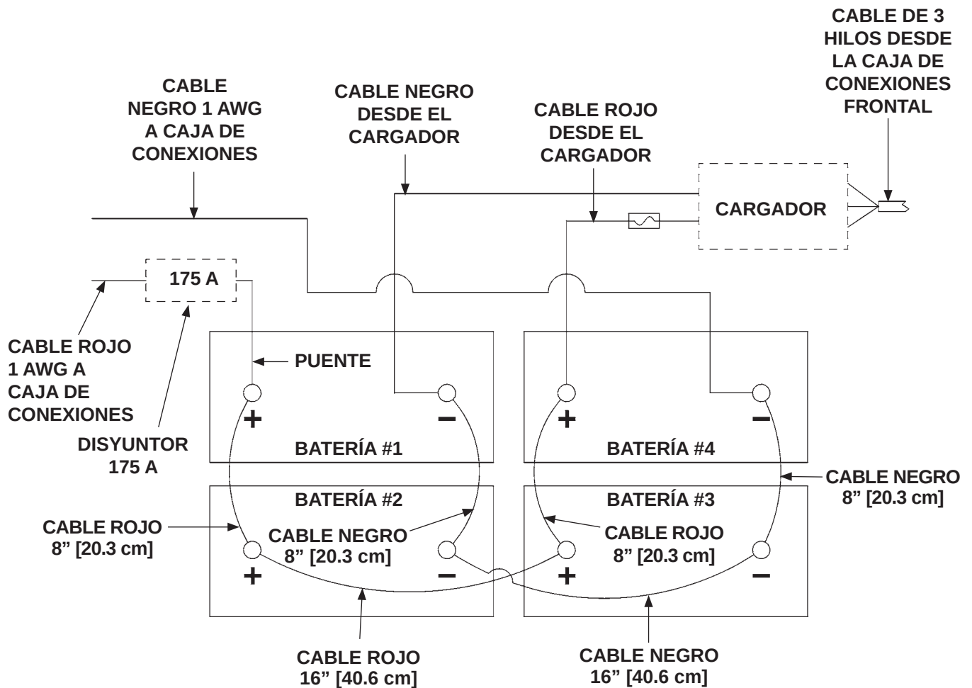
CONEXIONES DE LA BATERÍA - CAJA CON 4 BATERÍAS (CON CARGADOR) FIG. 54-1
