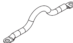
ENSAMBLE DEL CABLE NEGRO, CALIBRE 2, 8" [20.3 cm] DE LARGO N/P 251871-14 CANT. 2
