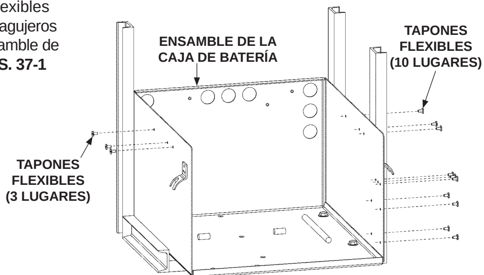
INSTALE LOS TAPONES FLEXIBLES (CAJA CON 2 BATERÍAS) FIG. 37-1
