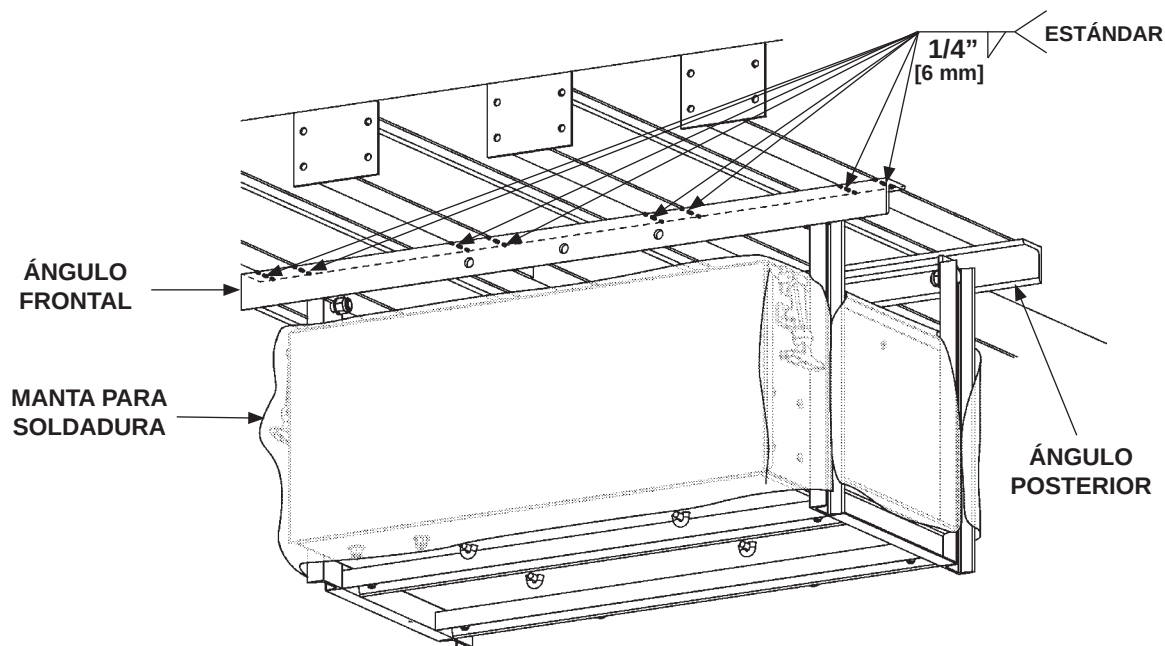
SOLDAR ENSABLE DE LA CAJA DE BATERÍA (SE MUESTRA CAJA CON 4 BATERÍAS) FIG. 41-1
