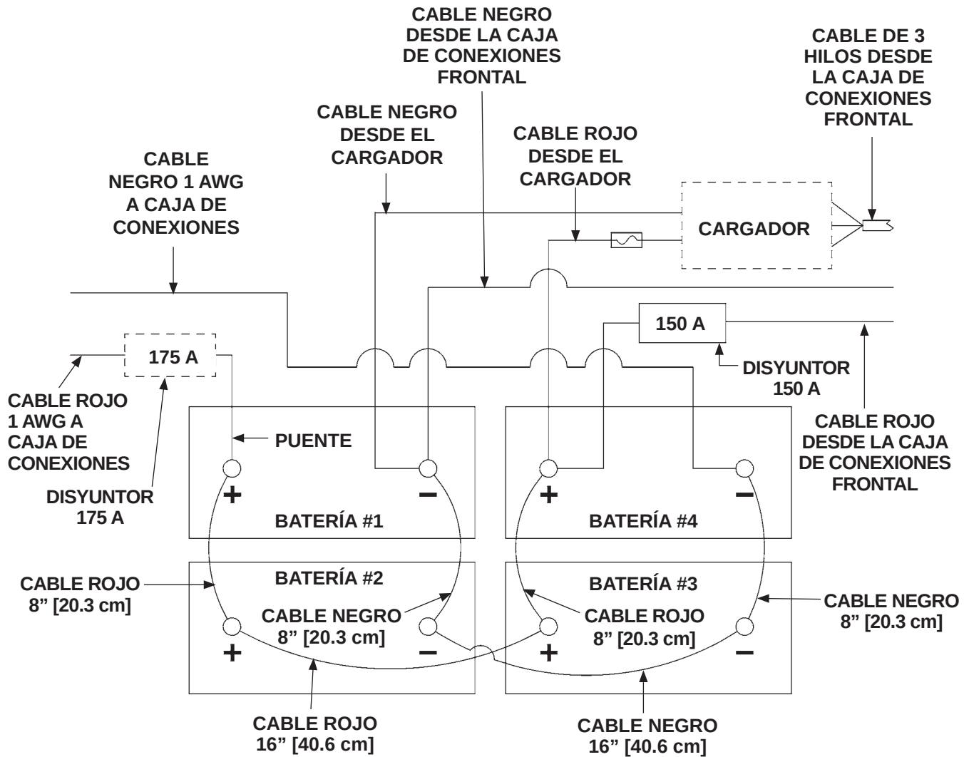
CONEXIONES DE LA BATERÍA - CAJA CON 4 BATERÍAS (CON CARGA DIRECTA Y CARGADOR)
