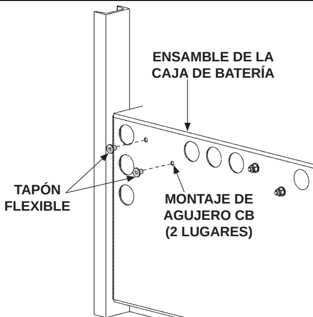
COLOCANDO LOS TAPONES DEL MONTAJE DE AGUJEROS CB (CAJA CON 2 BATERÍAS) FIG. 38-1
