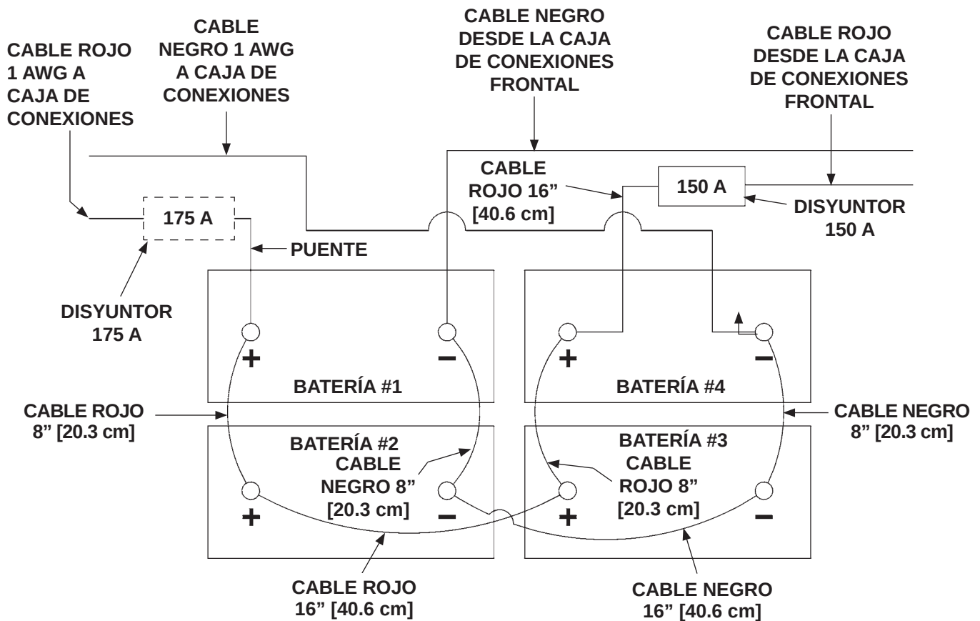
CONEXIONES DE LA BATERÍA - CAJA CON 4 BATERÍAS (CON CARGA DIRECTA) FIG. 53-1
