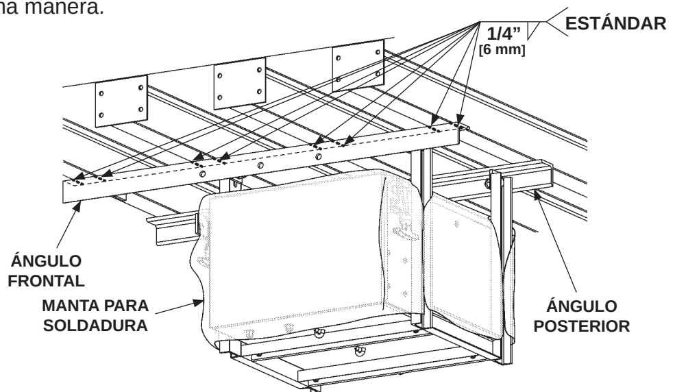
SOLDAR ENSABLE DE LA CAJA DE BATERÍA (SE MUESTRA CAJA CON 2 BATERÍAS) FIG. 40-1
