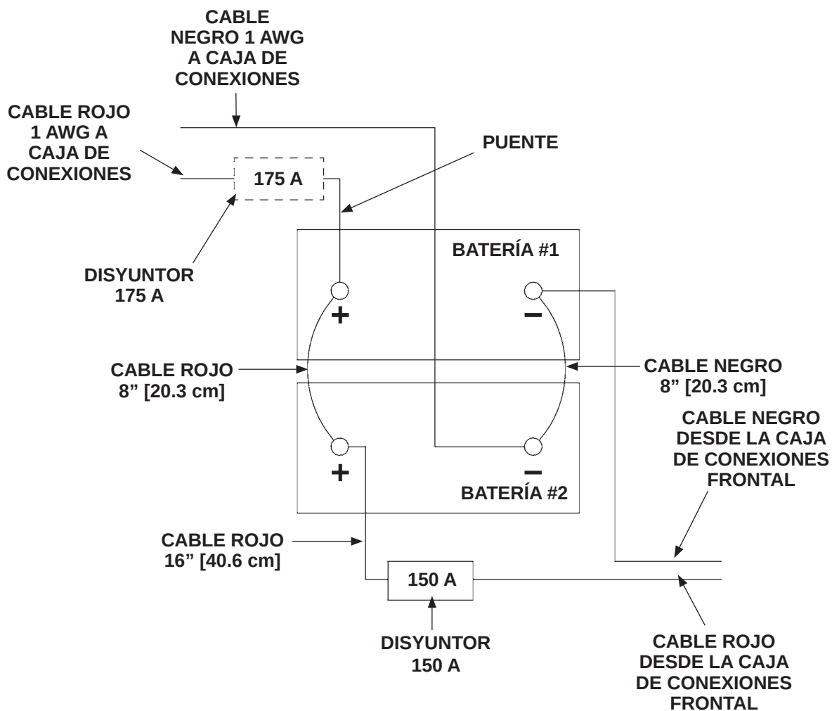
CONEXIONES DE LA BATERÍA - CAJA CON 2 BATERÍAS (CON CARGA DIRECTA) FIG. 50-1
