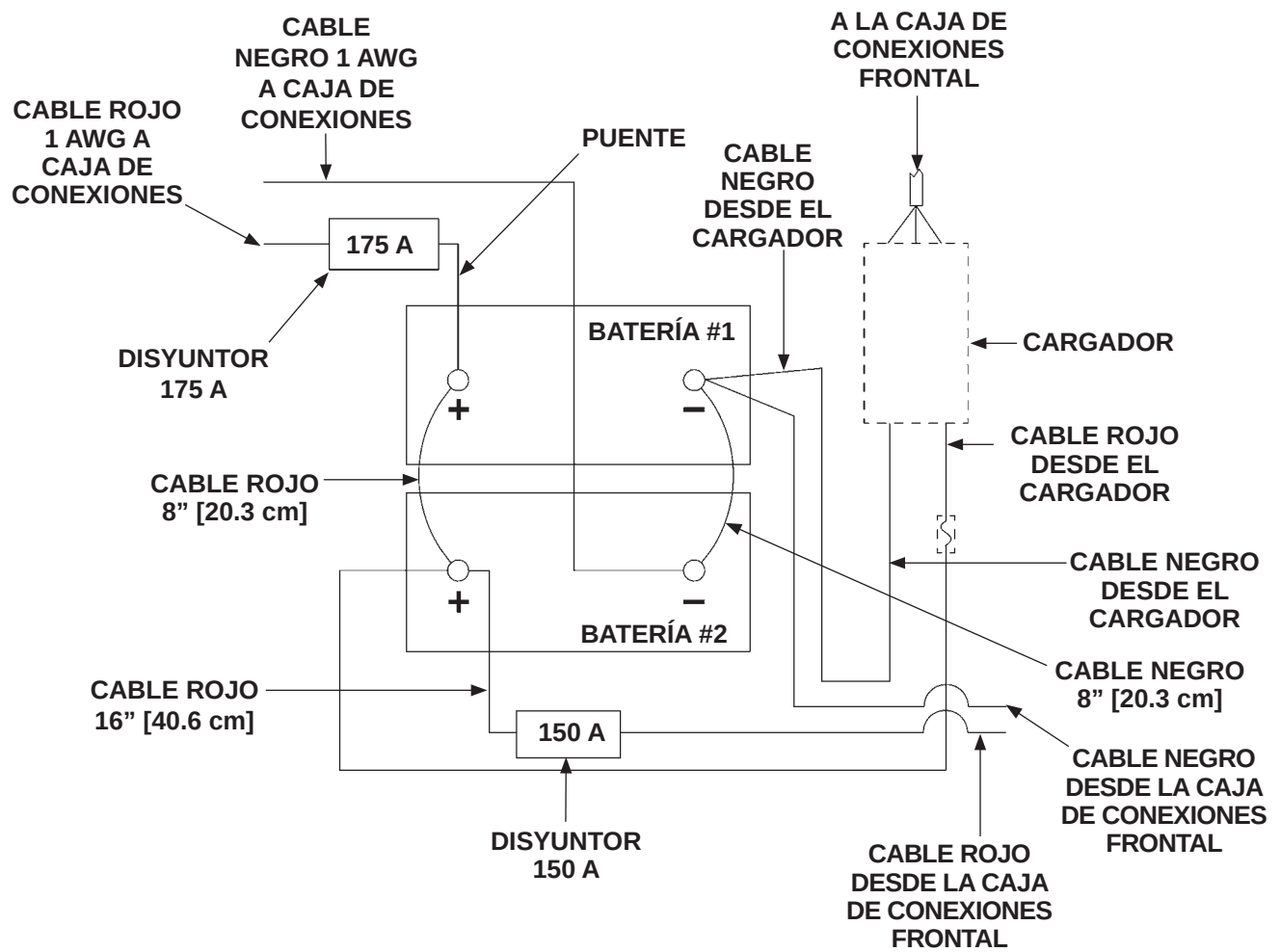
CONEXIONES DE LA BATERÍA - CAJA CON 2 BATERÍAS (CON CARGA DIRECTA Y CARGADOR)
