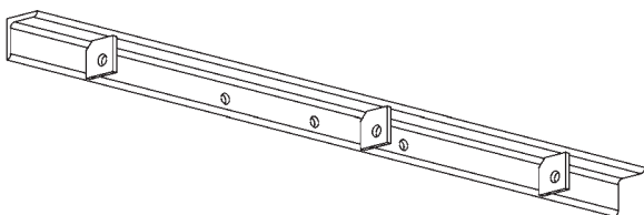
SOLDADURA DE ÁNGULO, CAJA DE BATERÍA, MONTAJE REMOTO, FRONTAL N/P 289538-01 CANT. 1
