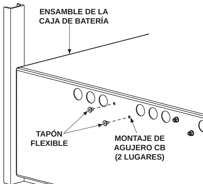
COLOCANDO LOS TAPONES DEL MONTAJE DE AGUJEROS CB (CAJA CON 4 BATERÍAS) FIG. 38-2
