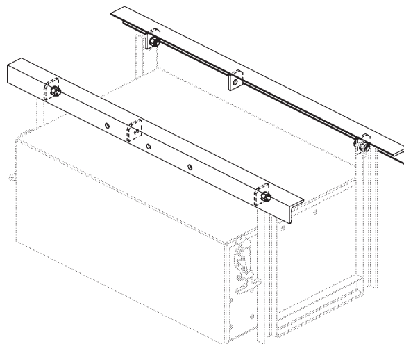
KIT DE MONTAJE PARA CAJA DE BATERÍA REMOTA N/P 287585-02 (SE MUESTRA CAJA DE 4 BATERÍAS) CANT. 1
