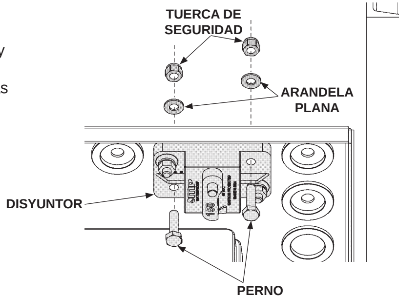
MONTAR EL DISYUNTOR (CAJA CON 2 BATERÍAS) FIG. 43-1
