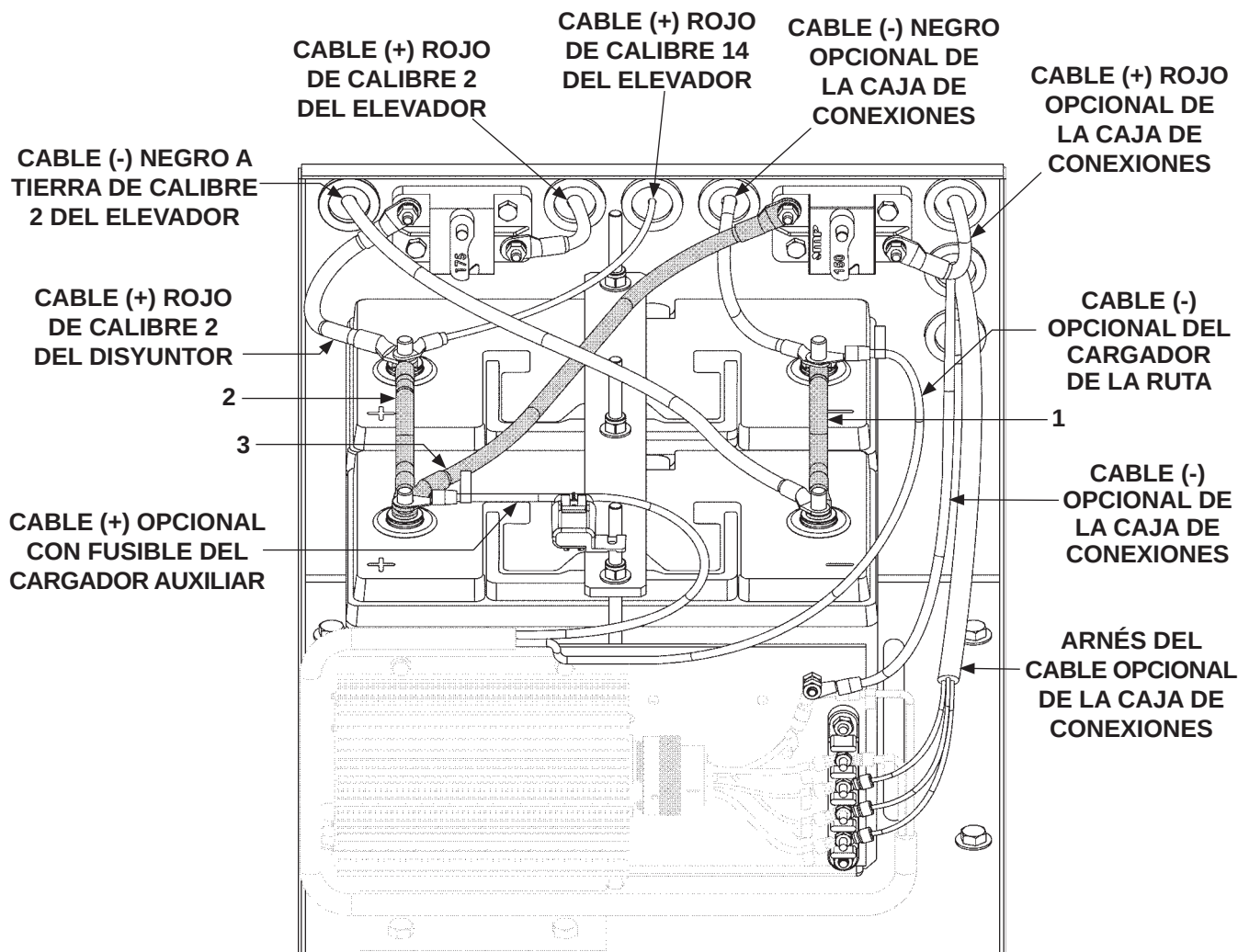
CONEXIONES DE LA BATERÍA DE 12 VOLTIOS (CAJA CON 2 BATERÍAS)
