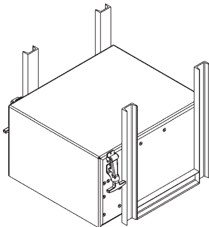
ENSAMBLE DE LA CAJA CON 2 BATERÍAS
