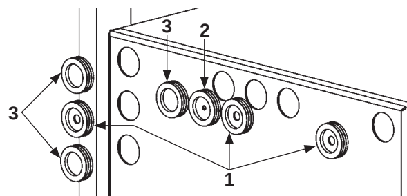
UBICACIONES DEL OJAL DE CAUCHO PARA EL KIT N/P 289690-03 FIG. 45-3
