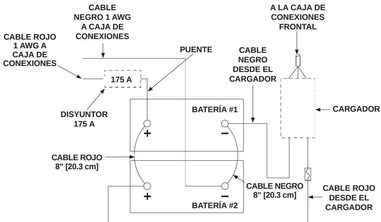
CONEXIONES DE LA BATERÍA - CAJA CON 2 BATERÍAS (CON CARGADOR, SIN CARGA DIRECTA)
