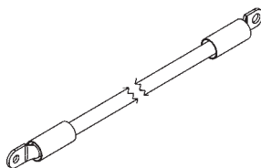
ENSAMBLE DEL CABLE ROJO, CALIBRE 2, 16" [40.6 cm] DE LARGO N/P 269308-16 (KITS 289690-01 Y 289690-02) CANT. 1
