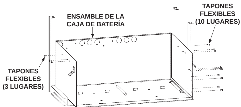
INSTALE LOS TAPONES FLEXIBLES (CAJA CON 4 BATERÍAS) FIG. 37-2
