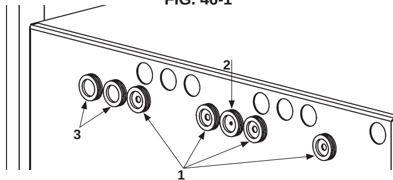
UBICACIONES DEL OJAL DE CAUCHO PARA EL KIT N/P 289690-12 FIG. 46-2
