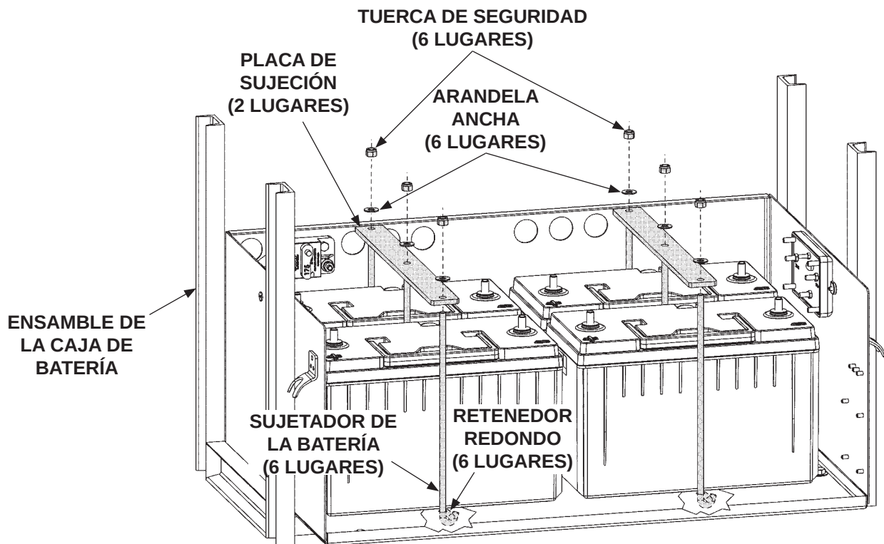
ASEGURAR LAS BATERÍAS (CAJA CON 4 BATERÍAS) FIG. 42-2
