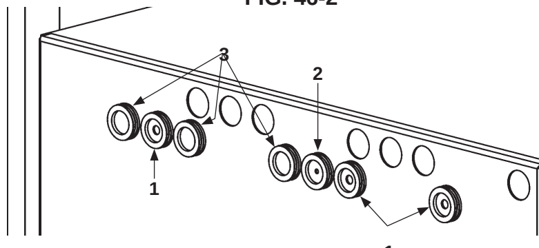
UBICACIONES DEL OJAL DE CAUCHO PARA EL KIT N/P 289690-13 FIG. 46-3
