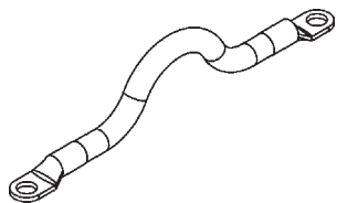
ENSAMBLE DEL CABLE ROJO, CALIBRE 2, 8" [20.3 cm] DE LARGO N/P 269308-10 CANT. 1
