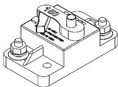
DISYUNTOR DE 150 A N/P 907207-02 (KITS 289690-01 Y 289690-02) CANT. 1
