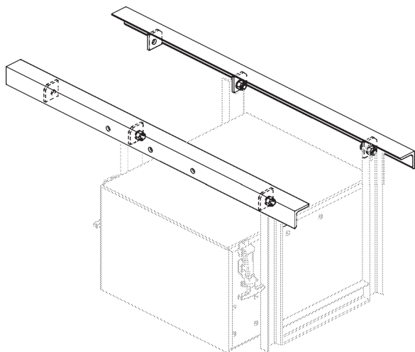
KIT DE MONTAJE PARA CAJA DE BATERÍA REMOTA N/P 287585-02 (SE MUESTRA CAJA DE 2 BATERÍAS) CANT. 1
