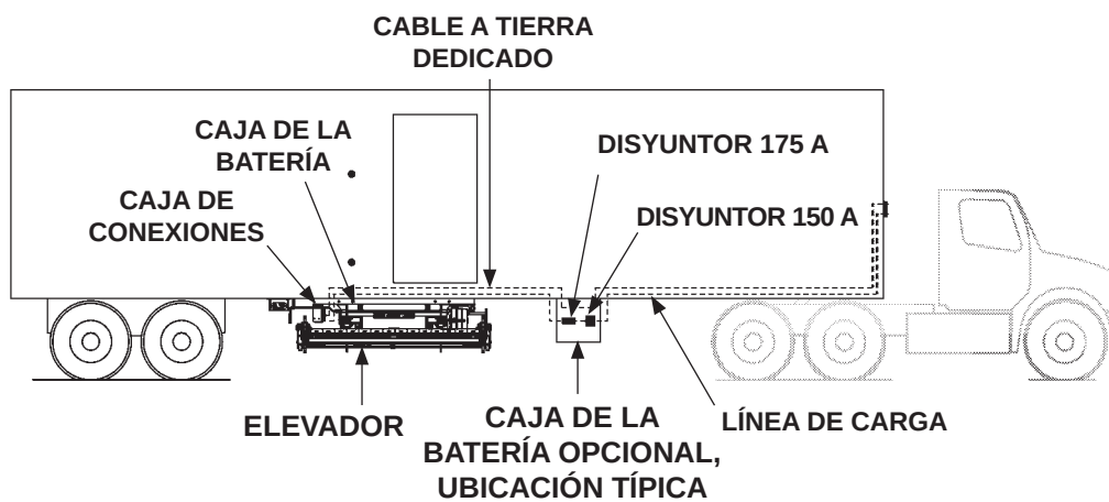
CAJA DE BATERÍA OPCIONAL INSTALADA EN TRÁILER (SE MUESTRA RA)
