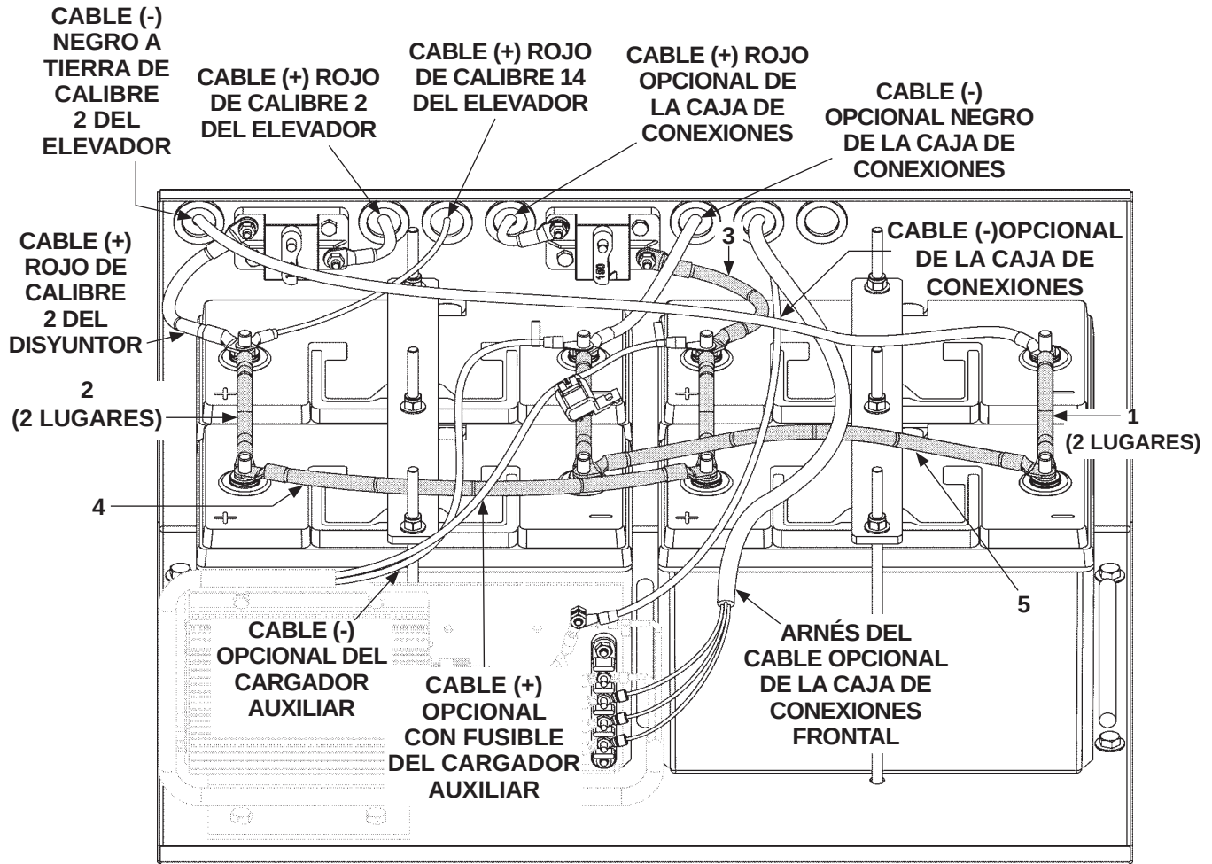
CONEXIONES DE LA BATERÍA DE 12 VOLTIOS (CAJA CON 4 BATERÍAS)
