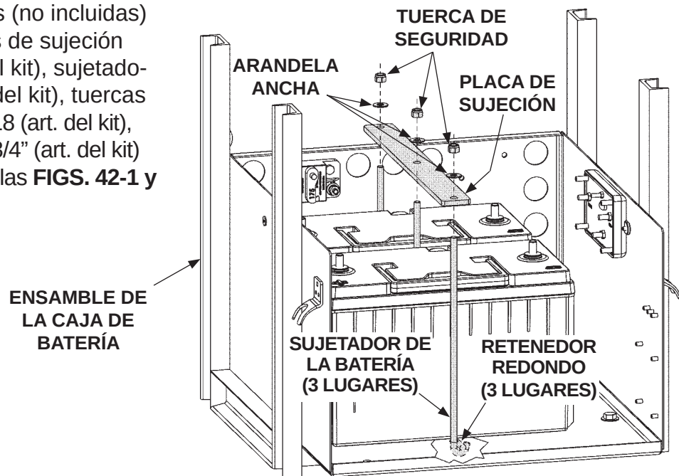
ASEGURAR LAS BATERÍAS (CAJA CON 2 BATERÍAS) FIG. 42-1
