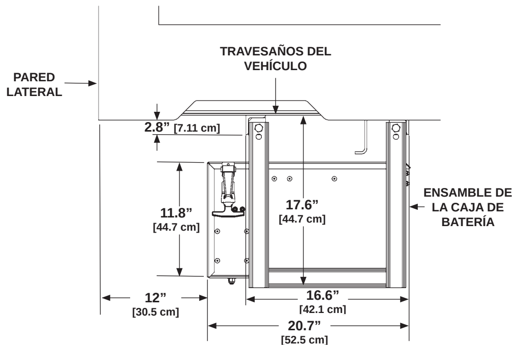
DIMENSIONES DE ESPACIO LIBRE DEL ENSAMBLE DE LA CAJA DE BATERÍA FIG. 39-2
