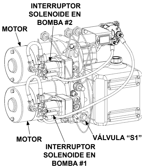
UNIDAD DE PODER CON BOMBA DUAL FIG. 28-1
