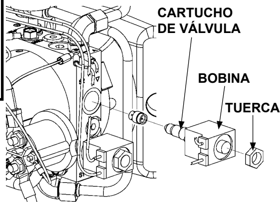
RETIRAR VÁLVULA SOLENOIDE FIG. 38-2
