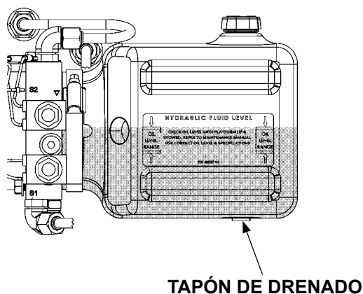
UNIDAD DE PODER FIG. 16-2
