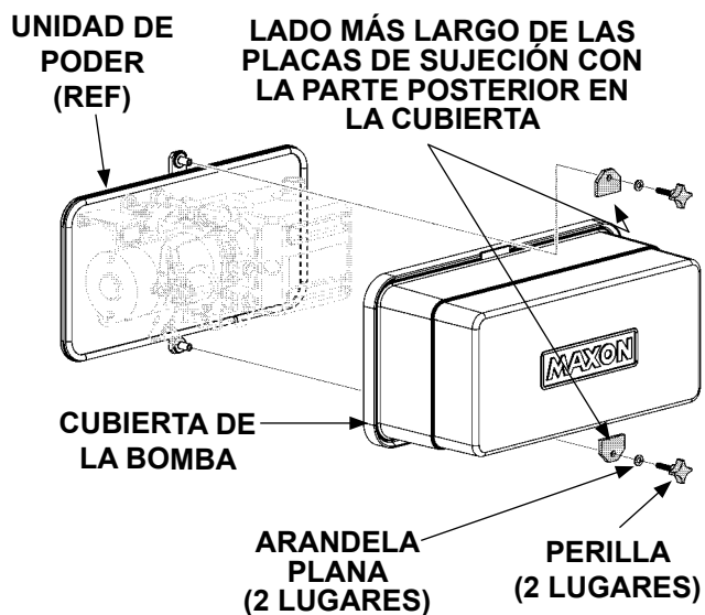
QUITAR LA CUBIERTA DE LA BOMBA FIG. 16-1
