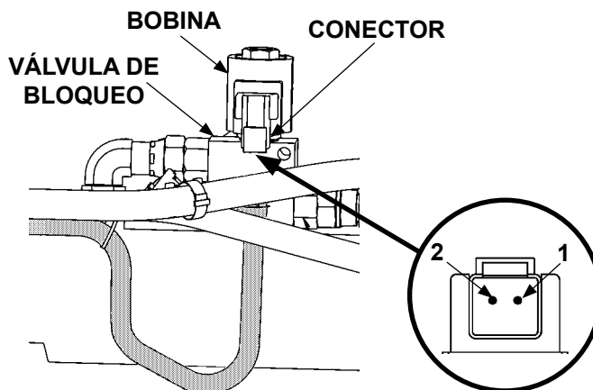
MEDIR LA RESISTENCIA DE BOBINA
