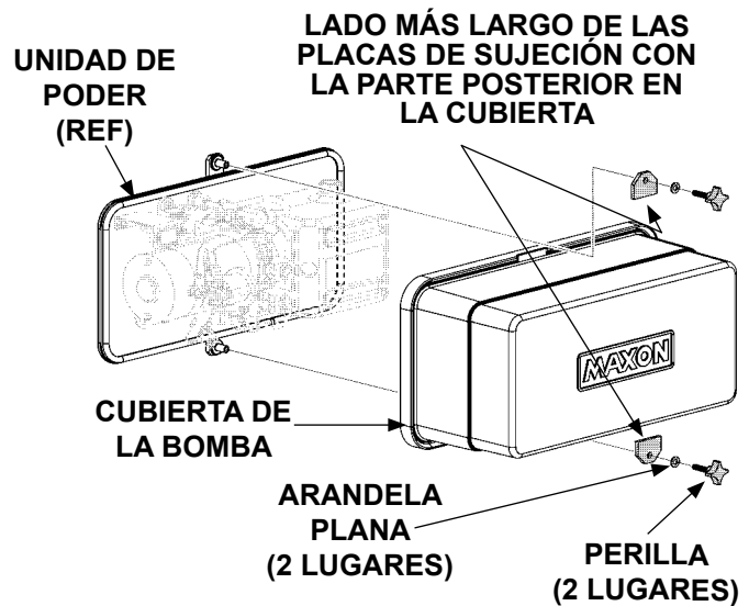
RETIRAR/INSTALAR LA CUBIERTA DE LA BOMBA
