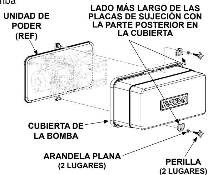
RETIRAR CUBIERTA DE LA BOMBA FIG. 47-3
