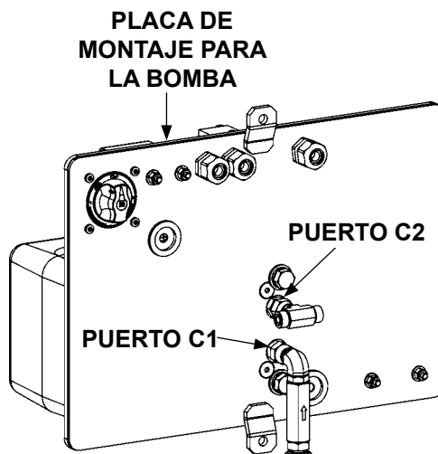
UNIDAD DE PODER CON BOMBA DUAL - VISTA POSTERIOR FIG. 28-2
