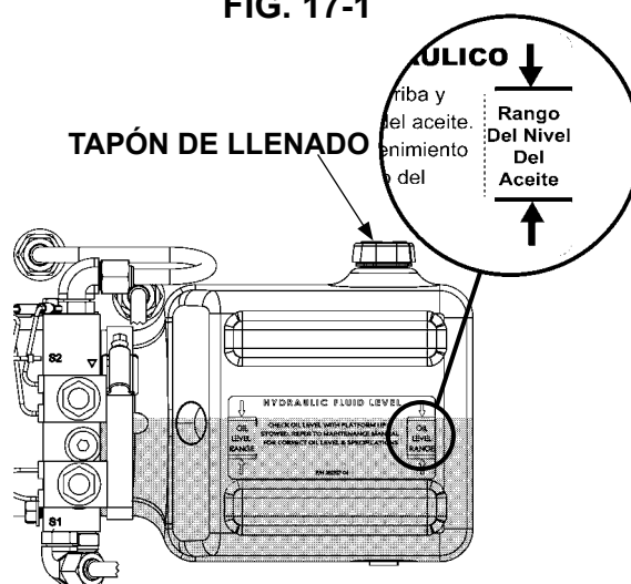
UNIDAD DE PODER FIG. 17-2
