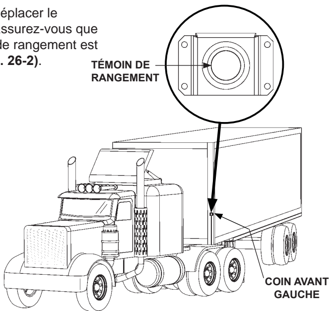
AVANT DE LA REMORQUE FIG. 26-2
