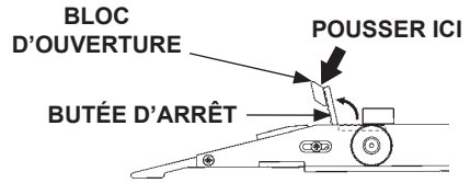
OUVRIR LES BUTÉES D'ARRÊT (VUE DROITE DE L'ÉLÉMENT RABBATABLE) FIG. 35-1
