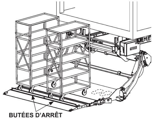
BUTÉES D'ARRÊT OUVERTES FIG. 35-2
