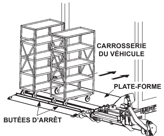
DÉCHARGER LA PLATE-FORME À HAUTEUR DE PLANCHER FIG. 35-3
