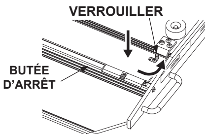
FERMETURE DES BUTÉES D'ARRÊT AVANT (VUE DROITE DE L'ÉLÉMENT RABATTABLE) FIG. 20-2
