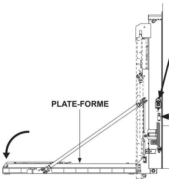
DÉPLIER LA PLATE-FORME FIG. 15-1
