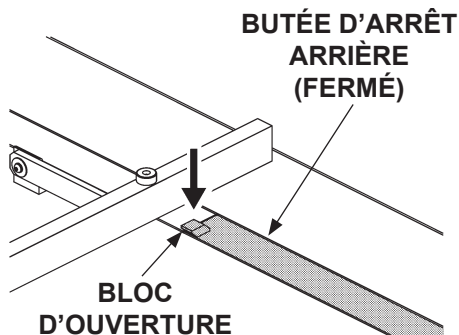
FERMETURE DE LA BUTÉE D'ARRÊT ARRIÈRE FIG. 20-1
