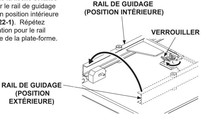
ROTATION DU RAIL DE GUIDAGE EN POSITION INTÉRIEURE (VUE DE LA PLATE-FORME CÔTÉ DROIT) FIG. 22-1
