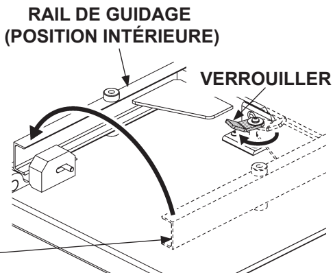
ROTATION DU RAIL DE GUIDAGE EN POSITION INTÉRIEURE (VUE DE LA PLATE-FORME CÔTÉ DROIT)
