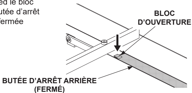
FERMETURE DE LA BUTÉE D'ARRÊT ARRIÈRE FIG. 27-2
