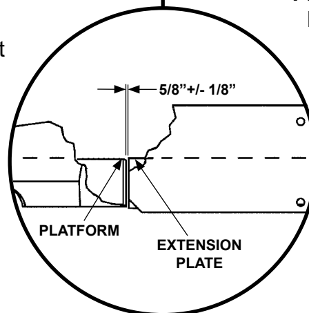
HORIZONTAL GAP FIG. 49-1B
