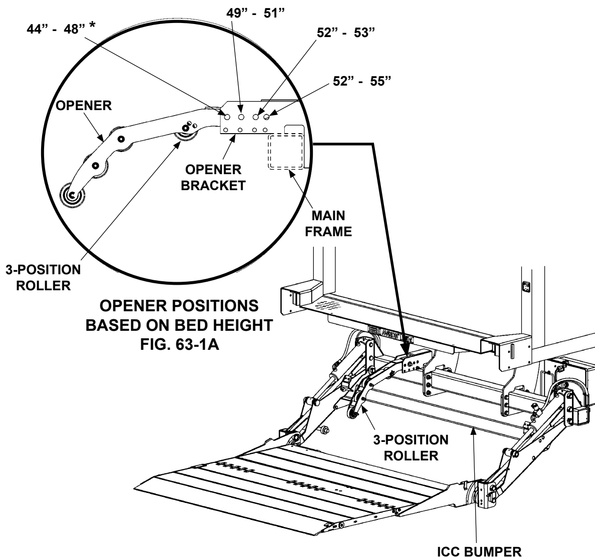
GPTLR-25 OR GPTLR-33 FIG. 63-1
