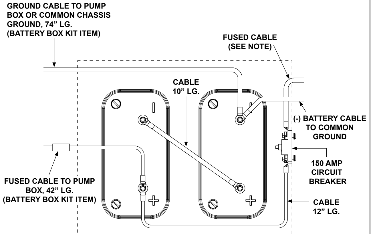
12 VOLT BATTERY CONNECTIONS FOR 24 VOLT POWER FIG. 31-1
