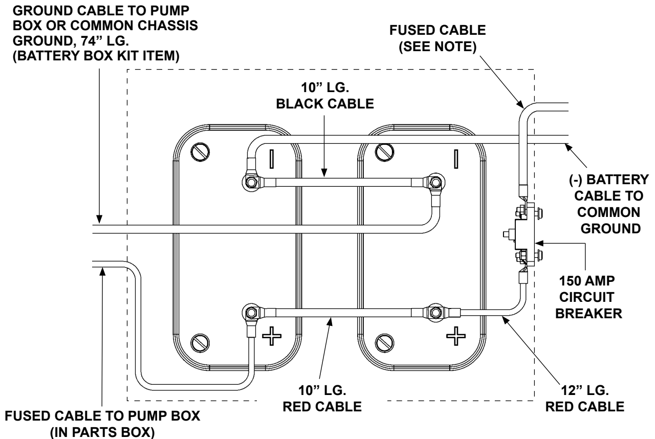
12 VOLT BATTERY CONNECTIONS FOR 12 VOLT POWER FIG. 30-1
