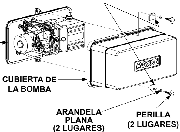
QUITAR LA CUBIERTA DE LA BOMBA FIG. 16-1
