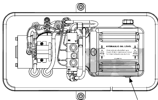
UNIDAD DE PODER FIG. 16-2
