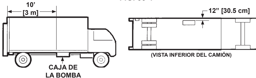
INSTALACIÓN USUAL PARA 10 PIES [3 m] FIG. 39-2
