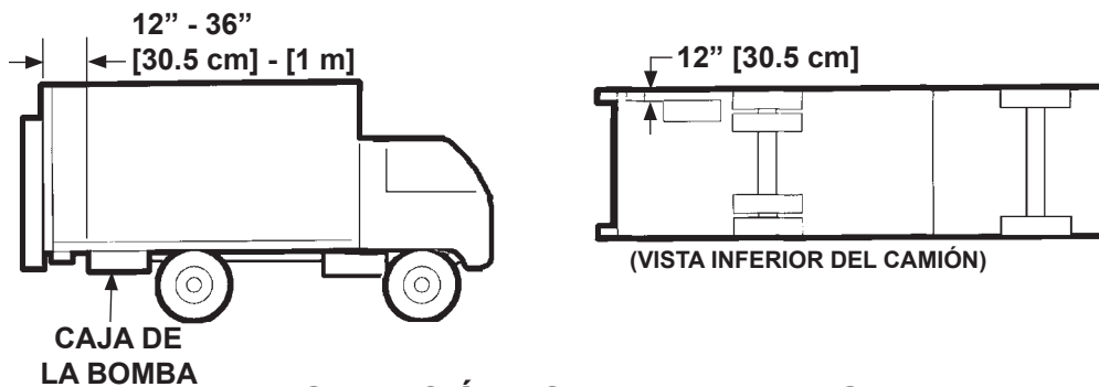
INSTALACIÓN USUAL PARA 3 PIES [1 m] FIG. 39-1
