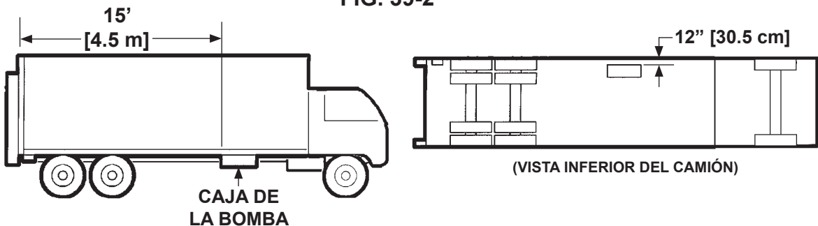
INSTALACIÓN USUAL PARA 15 PIES [4.5 m] FIG. 39-3
