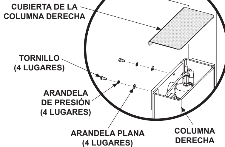
REINSTALAR CUBIERTA DE COLUMNA DERECHA FIG. 76-1A
